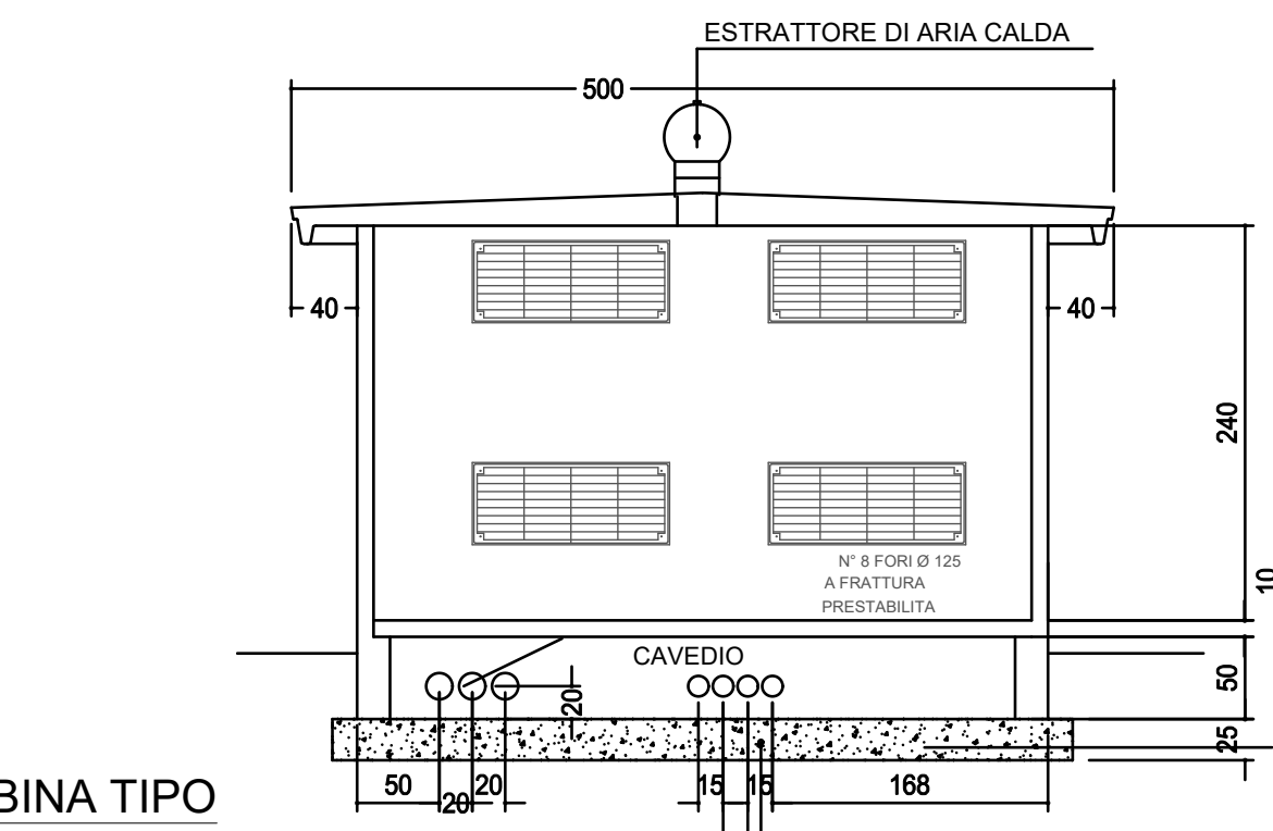
SEZIONE CABINA TIPO scala 1:50
