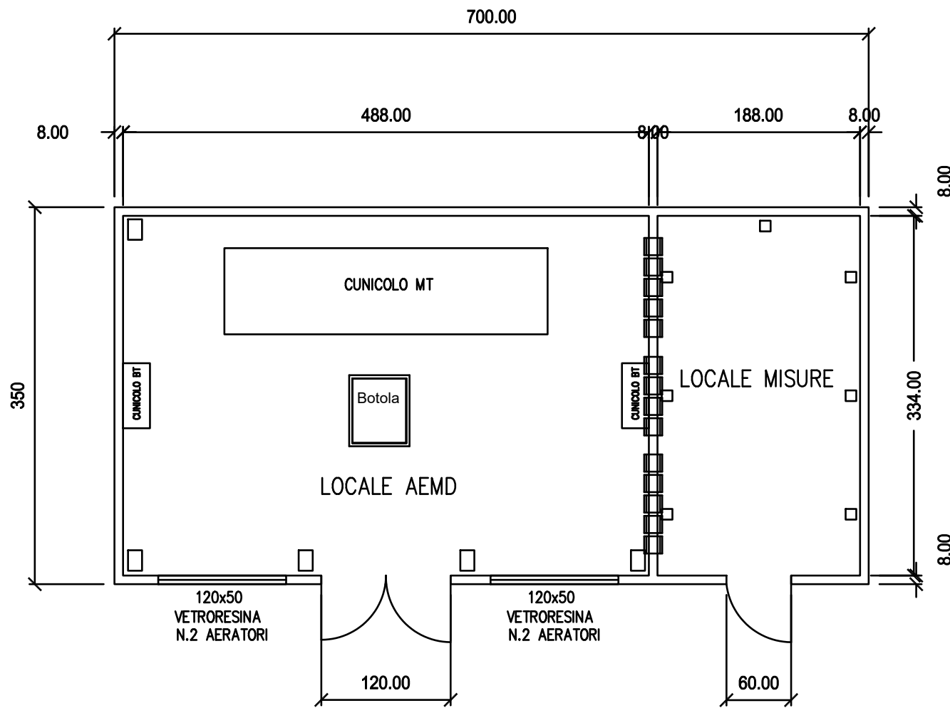
PIANTA CABINA TIPO scala 1:50
