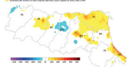
FIGURA 2a Anomalia del numero di notti tropicali dell'anno 2020 rispetto al clima 1961-1990
