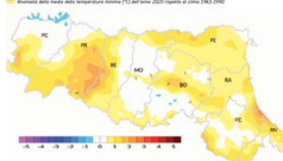
FIGURA 3 Anomalia della media della temperatura minima (°C) dell'anno 2020 rispetto al clima 1961-1990
