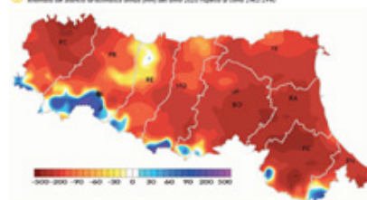
FIGURA 2b Anomalia del bilancio idroclimatico annuo (mm) dell'anno 2020 rispetto al clima 1961-1990
