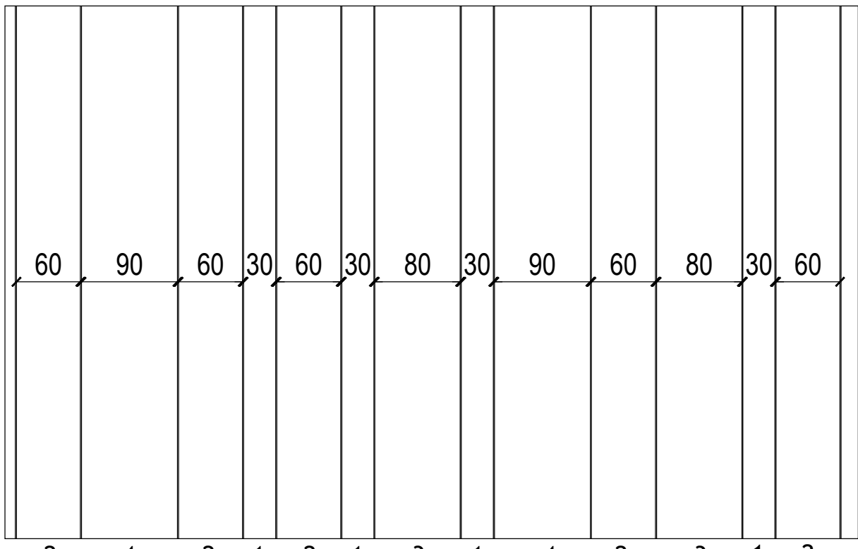
TESSITURA TIPO DELLA PAVIMENTAZIONE IN PIETRA ESISTENTE
