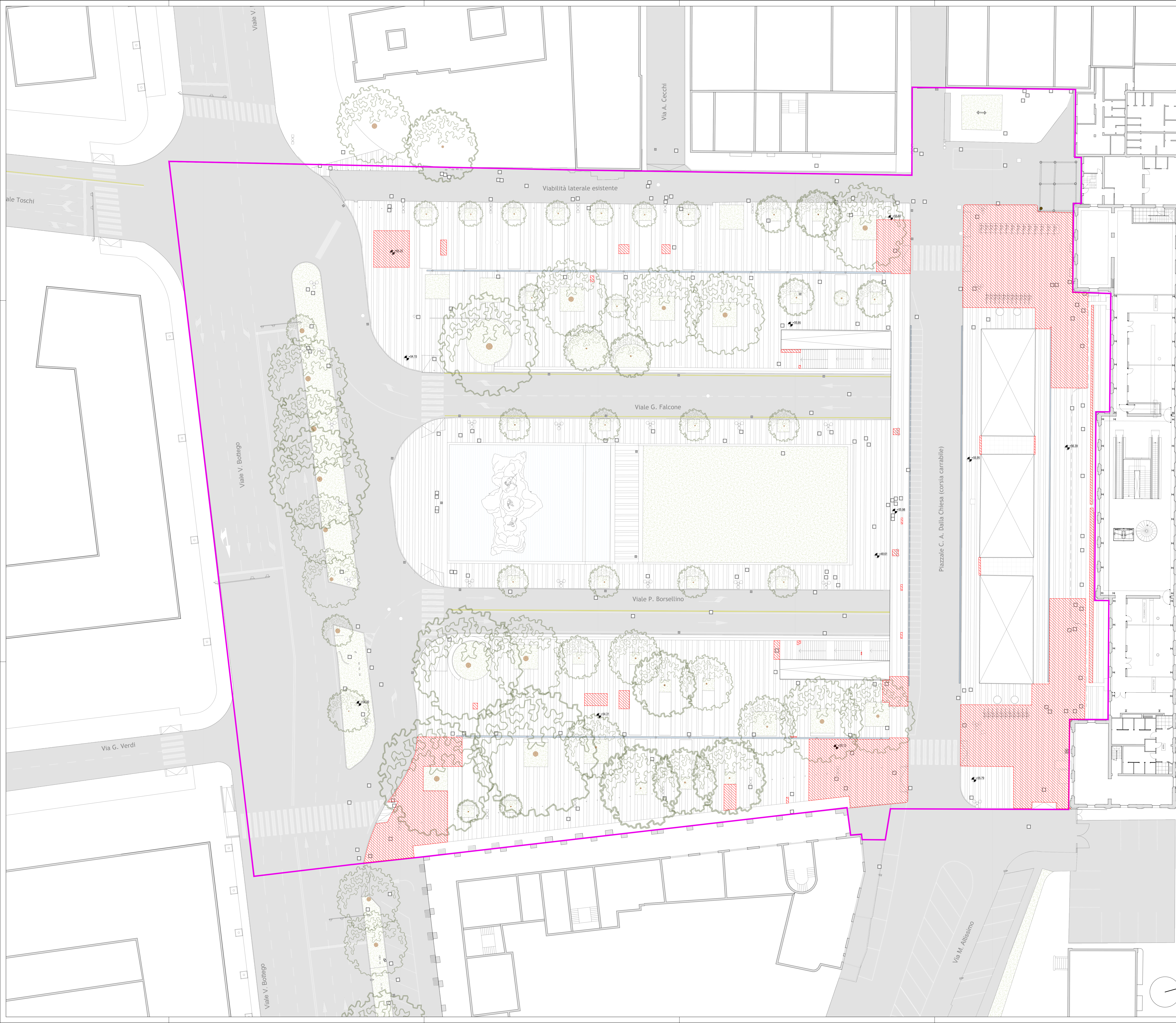
TESSITURA TIPO DELLA PAVIMENTAZIONE IN PIETRA ESISTENTE
