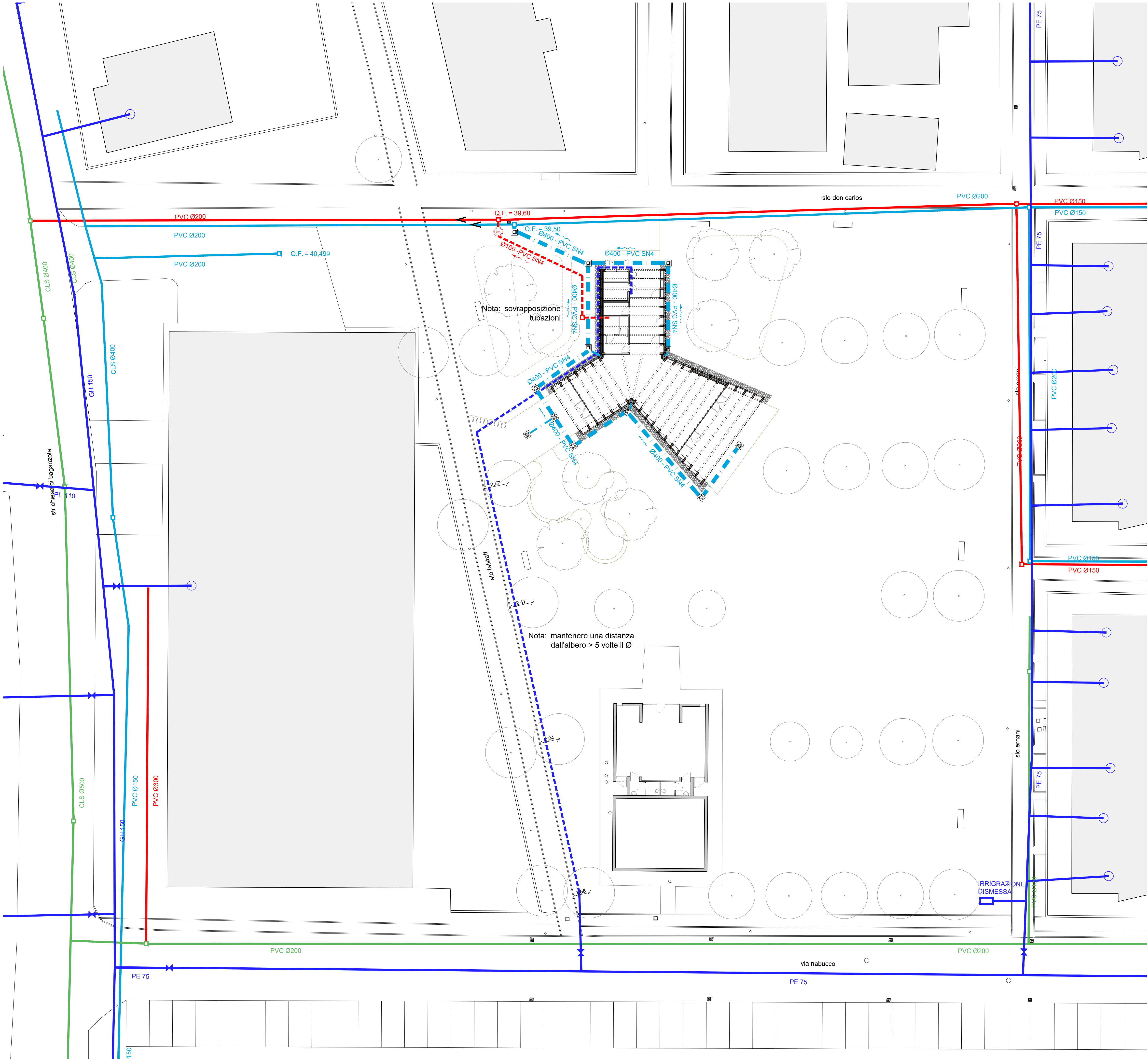
RETE FOGNARIA E RETE IDRICA - 1:200
