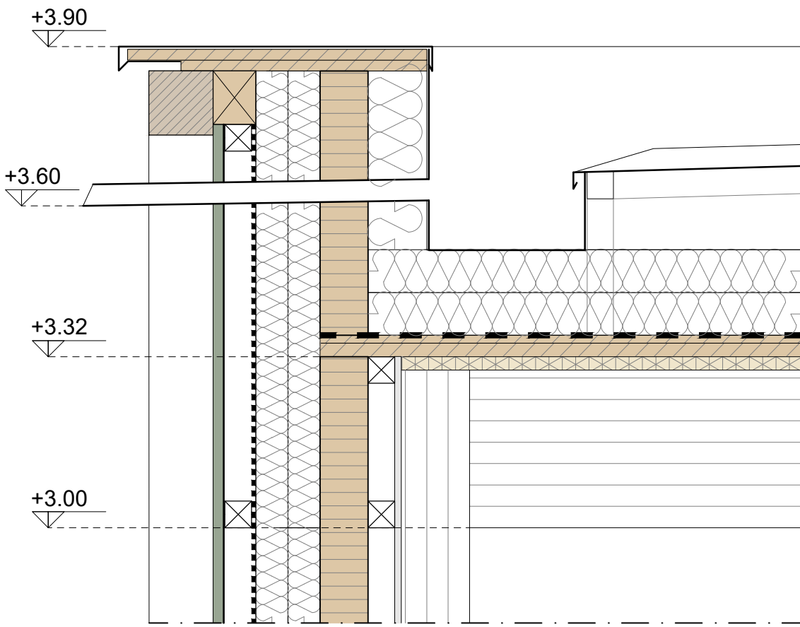
DETTAGLIO SEZIONE GRONDA E TROPPOPIENO Ø40 mm - 1:10
