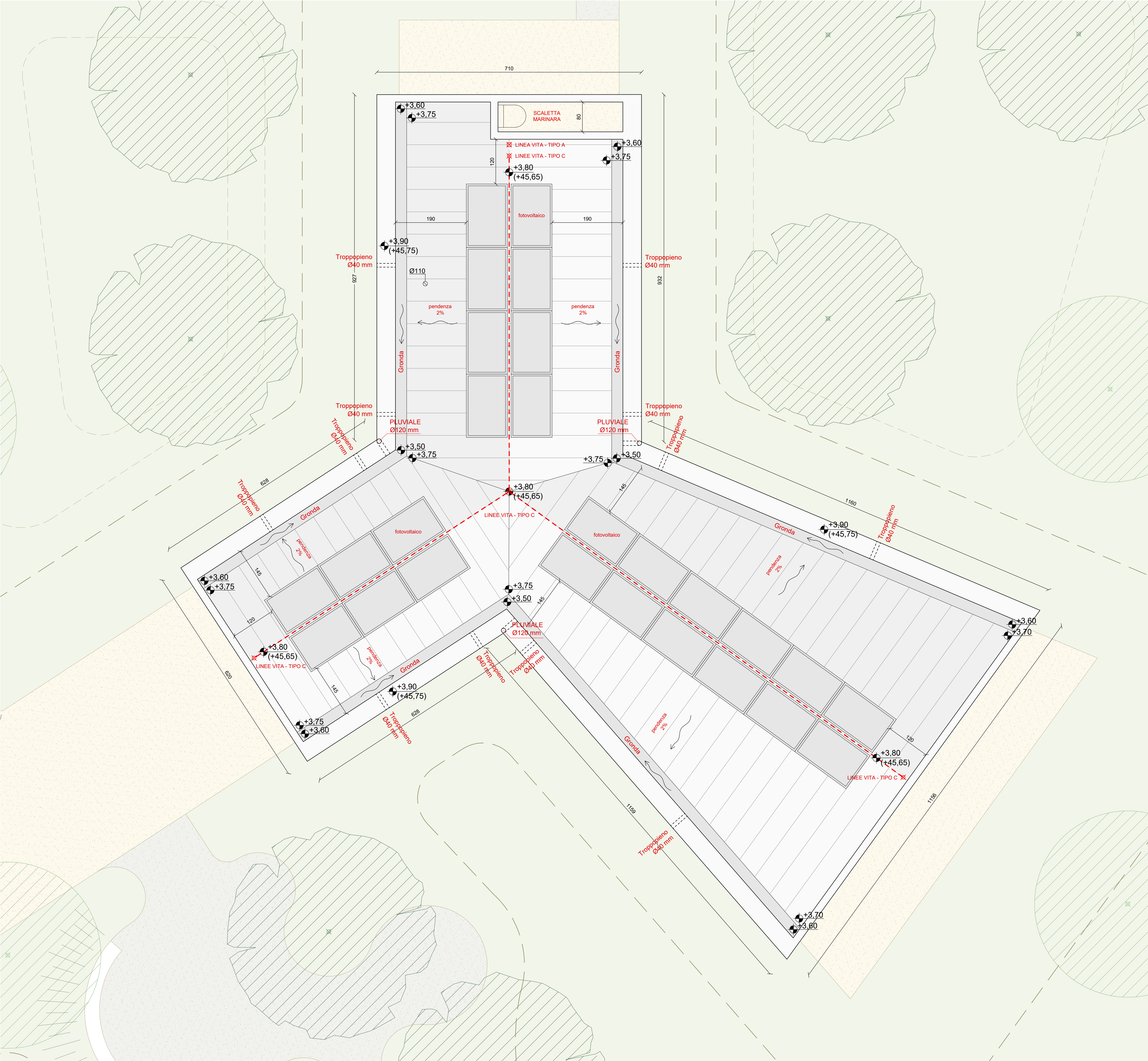
PIANTA DELLA COPERTURA - 1:50
