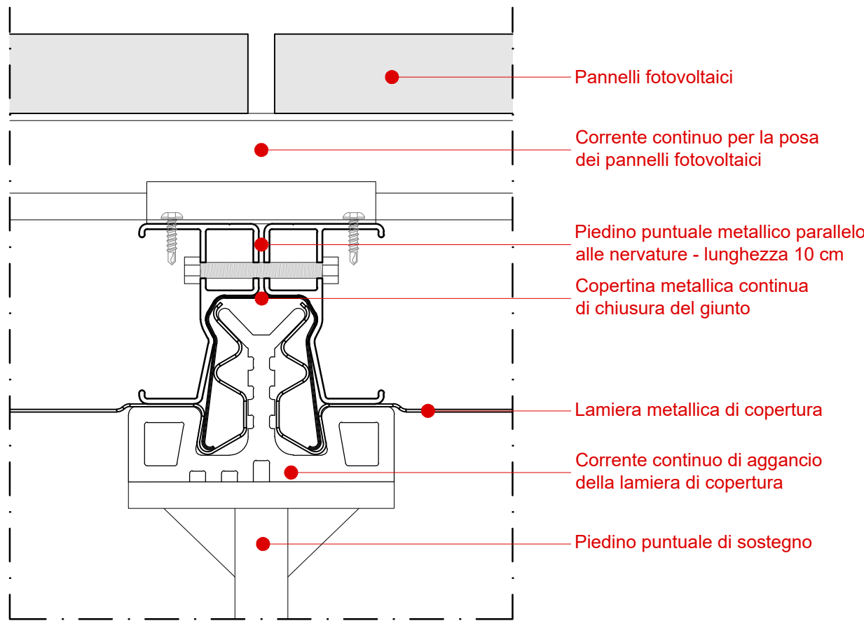
DETTAGLIO TIPO AGGANCIO FOTOVOLTAICO - 1:2
