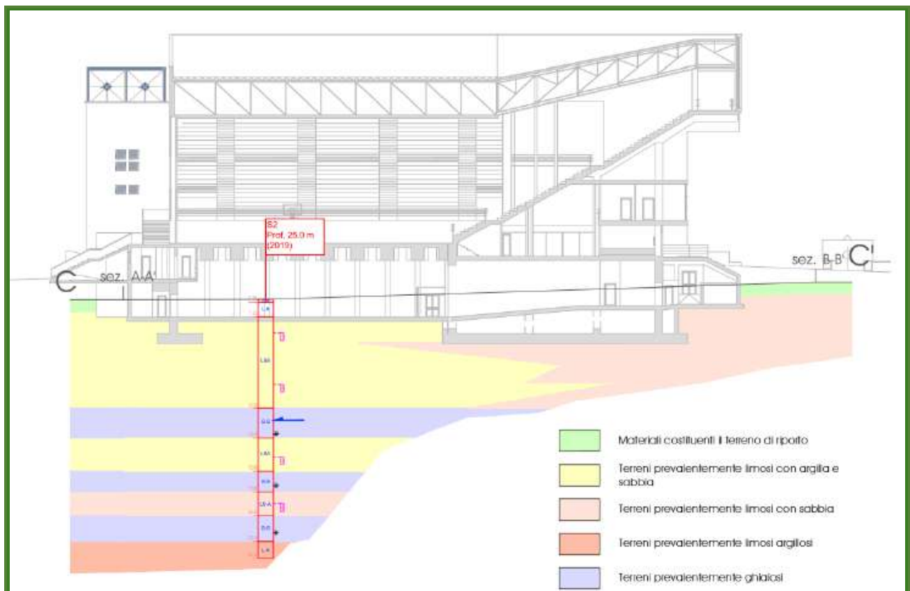
Figura 6 – Stratigrafia dei terreni dedotta dalla relazione geologica
