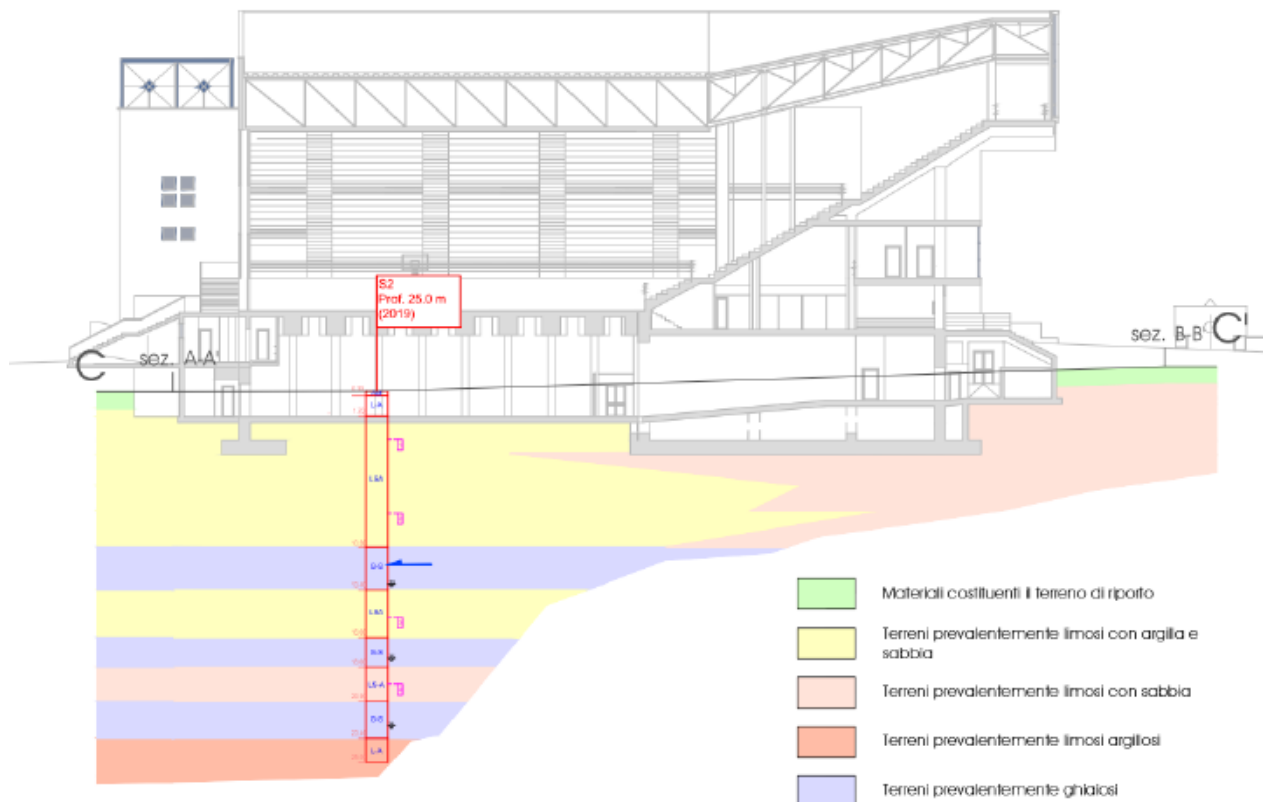
Figura 15: sezione litostratimetrica
