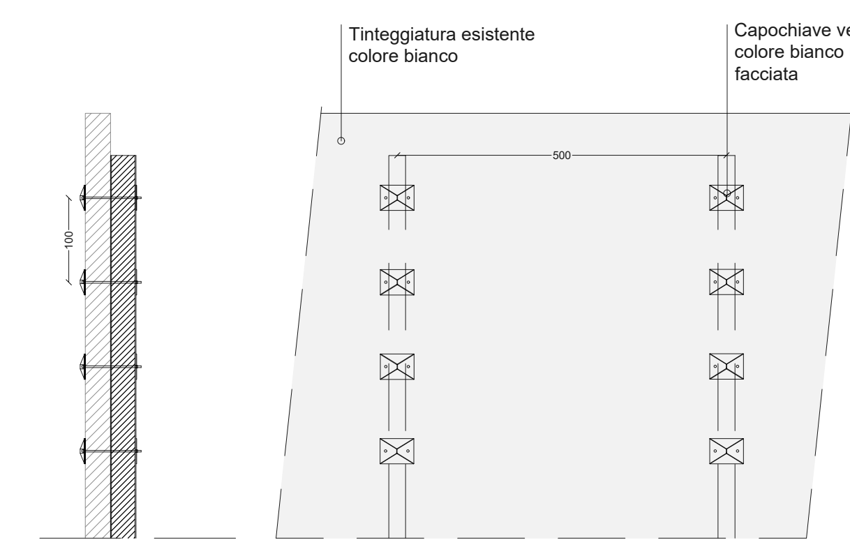
DETTAGLIO CAPOCHIAVE PARETI SCALE ESTERNE (tav. strutturale PFTE.ST06)
