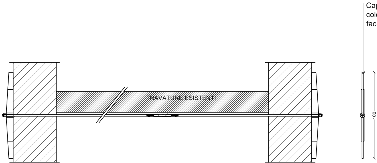
DETTAGLIO CAPOCHIAVE PARETI TORRE ( tav. strutturale PFTE.ST07)
