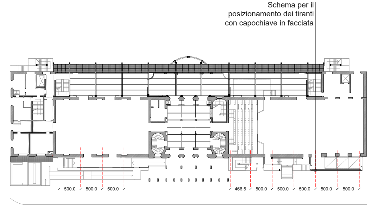
PIANTA II LIVELLO
