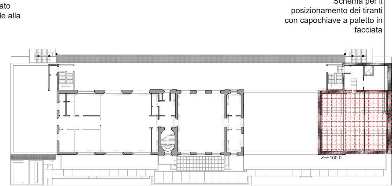
PIANTA IV LIVELLO
