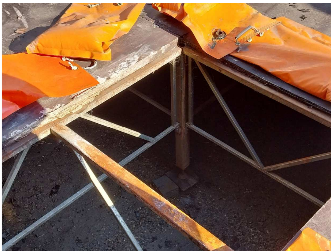
Arena Shakespeare – dettaglio struttura pavimentazione palcoscenico
