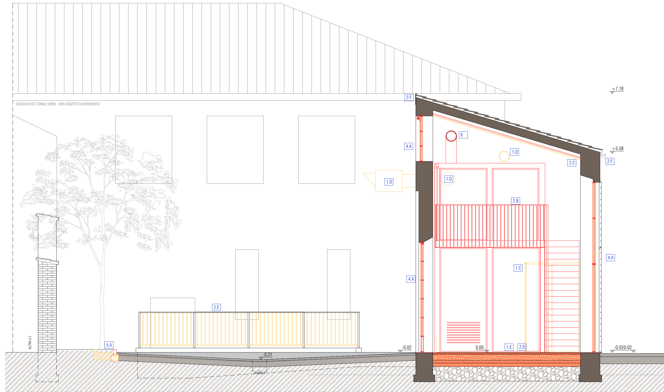
SEZIONE C-C
