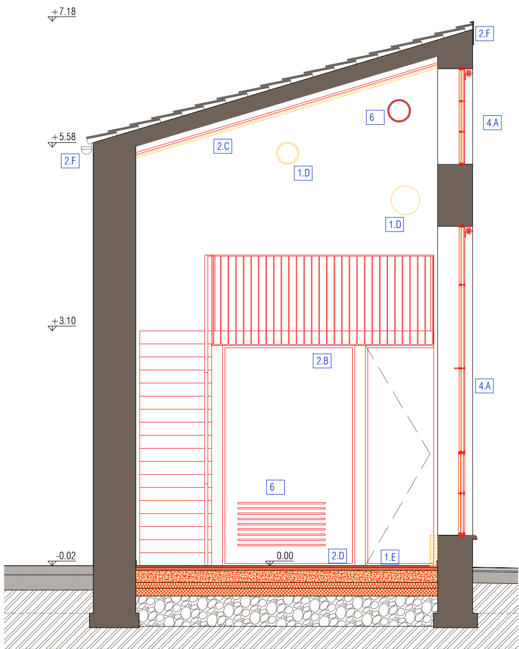
SEZIONE D-D
