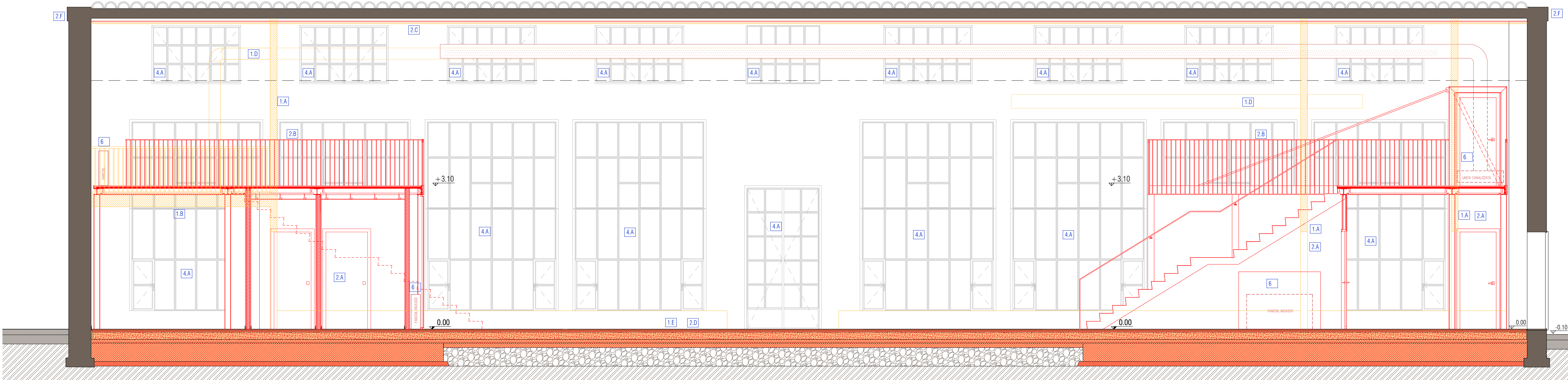
SEZIONE A-A
