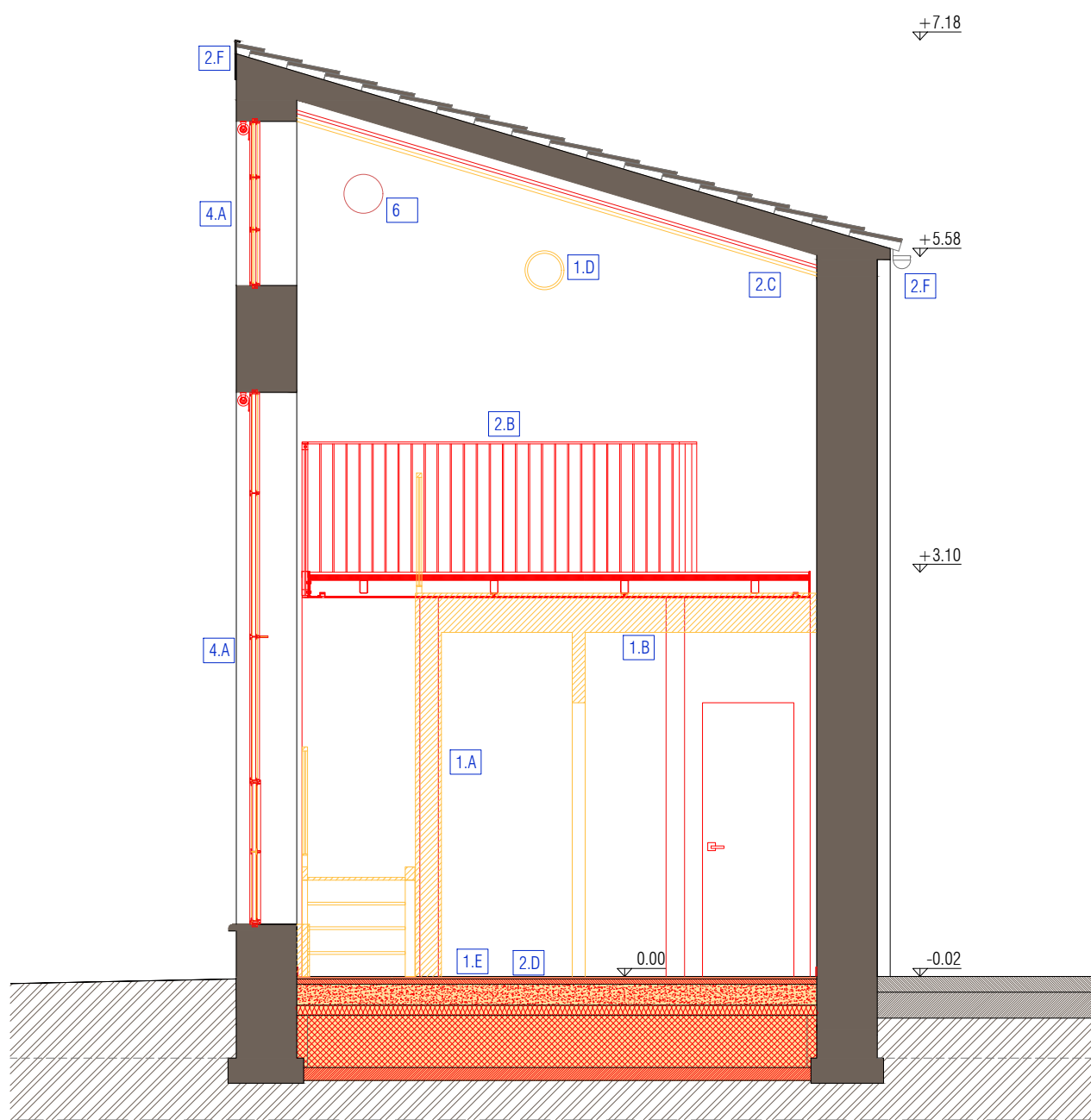
SEZIONE B-B
