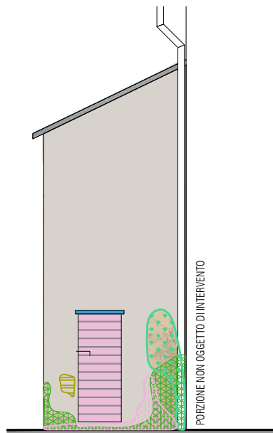
PROSPETTO OVEST
