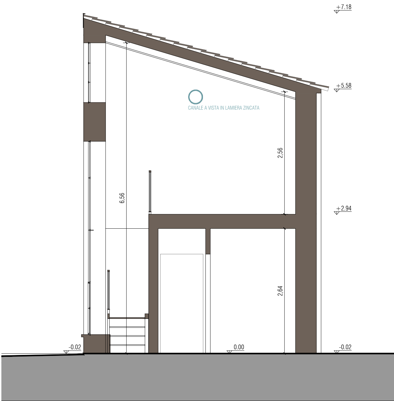
SEZIONE B-B
