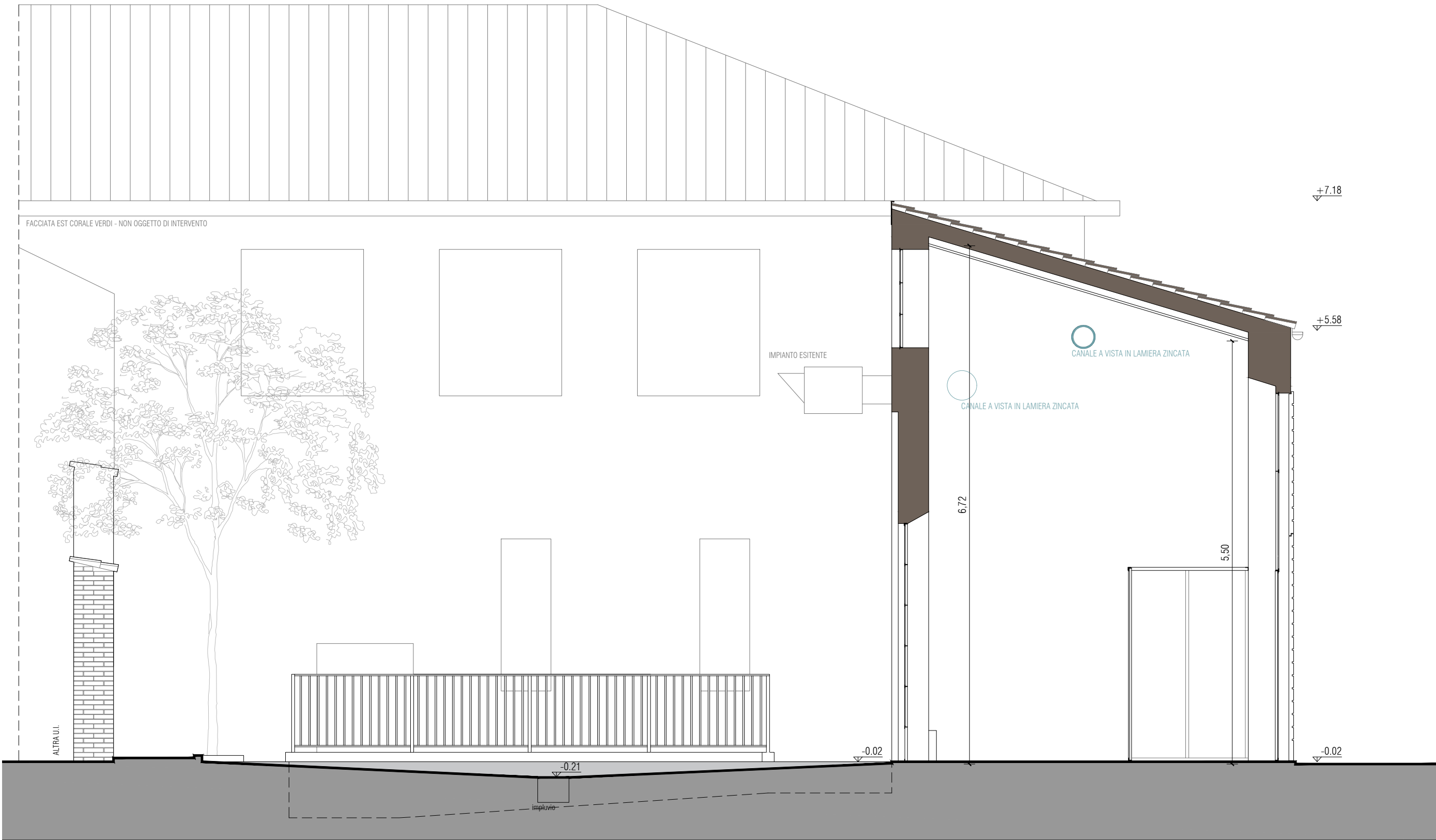
SEZIONE C-C
