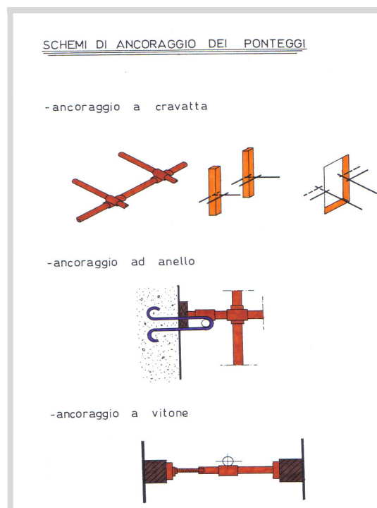
Figura 6. esempi di ancoraggi
