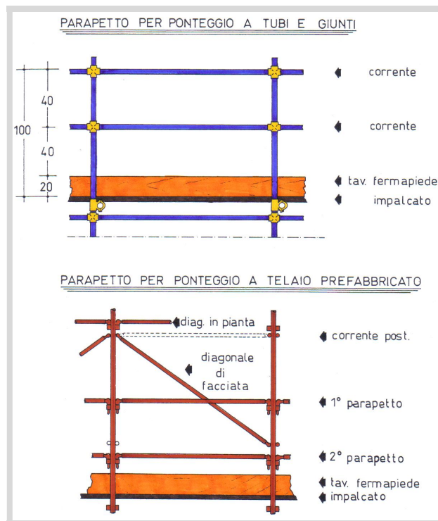
Figura 5. esempi di parapetti
