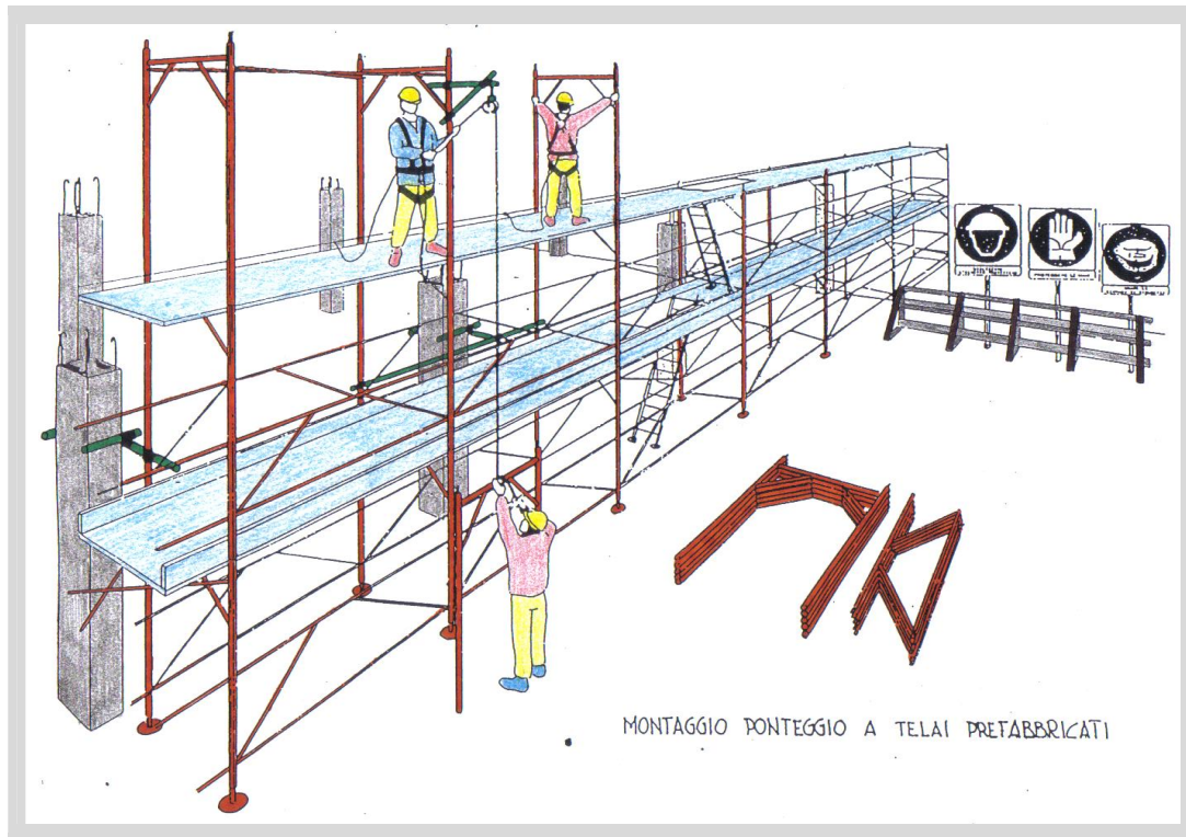
Figura 4. Esempio di corretta messa in opera di ponteggio a telai prefabbricati
