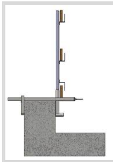
Figura 7. Tipologia parapetto
