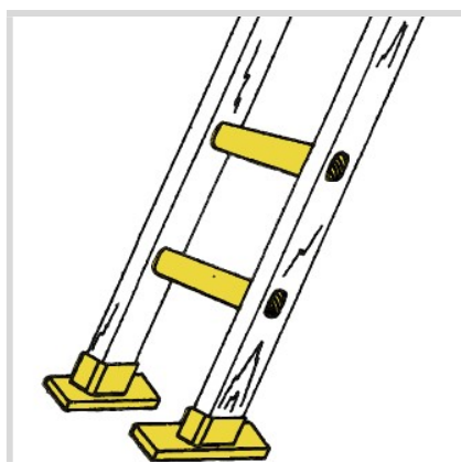
Figura 9: Le scale devono essere dotate di dispositivi antisdrucciolevoli alle estremità inferiori
