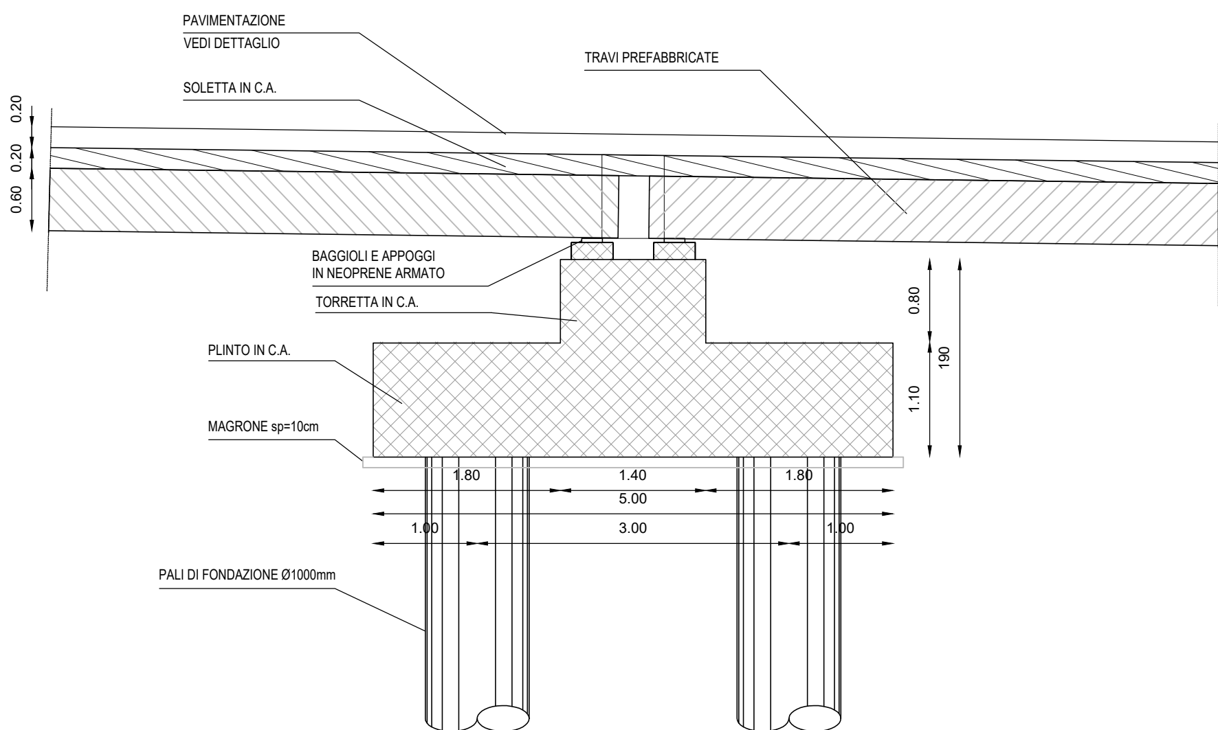
SEZIONE A-A
