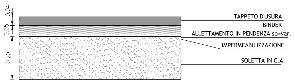
PACCHETTO STRADALE VIADOTTO Scala 1:10
