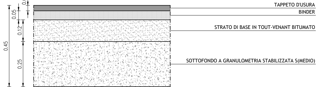
PACCHETTO STRADALE RILEVATO Scala 1:10
