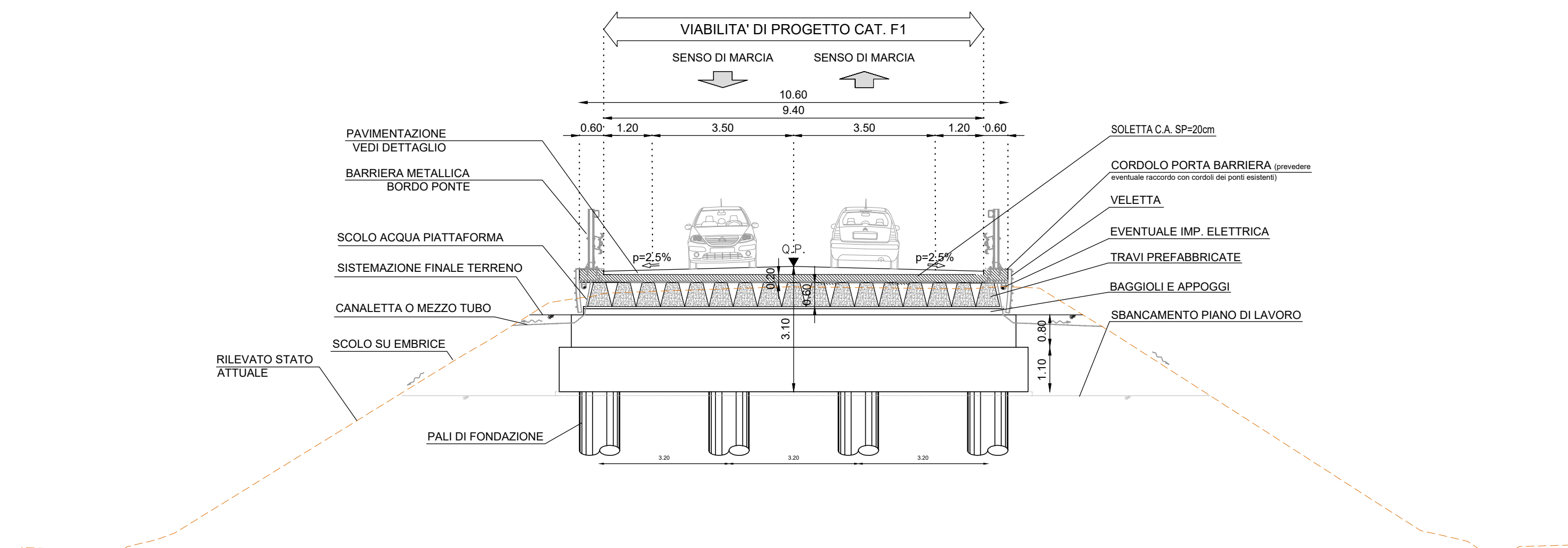
SEZIONE TIPO VIADOTTO IN CORRISPONDENZA DELLE PILE Scala 1:100
