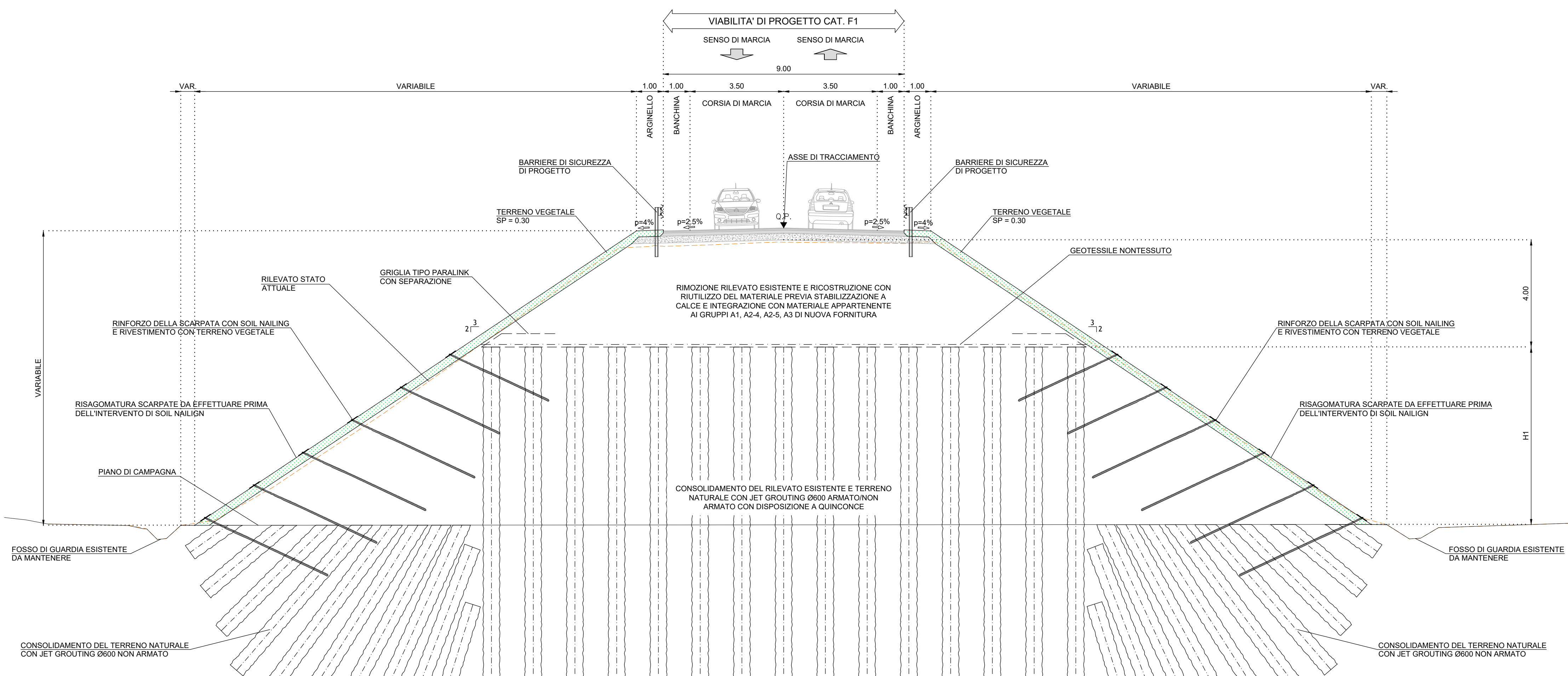
SEZIONE TIPO RILEVATO H>7m Scale 1:100
