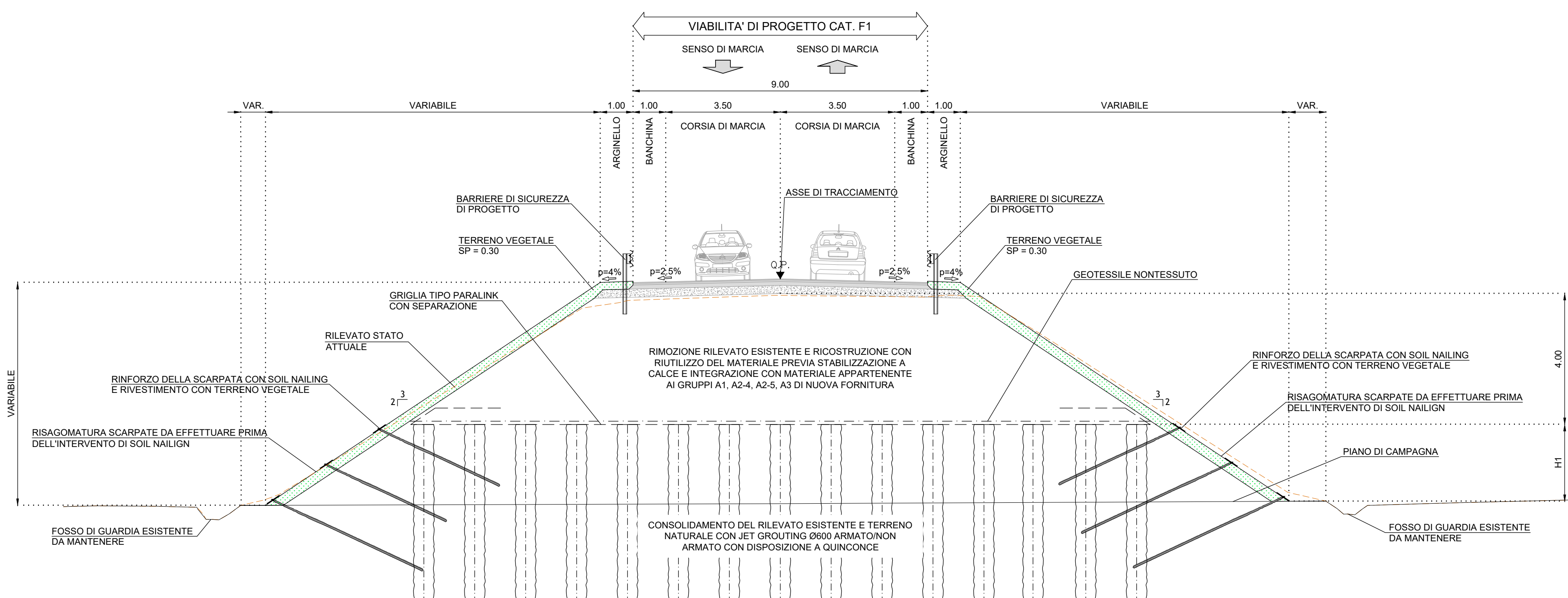
SEZIONE TIPO RILEVATO H>7m Scale 1:100
