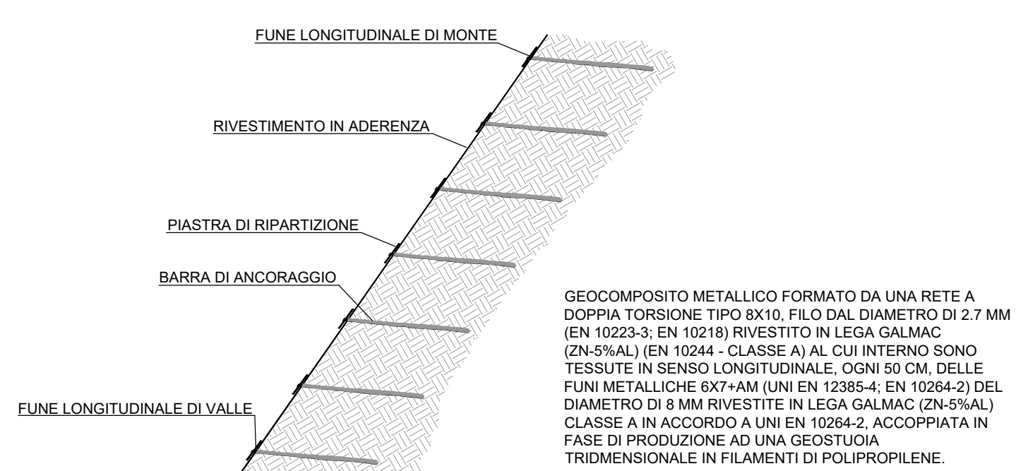
SEZIONE TIPO DELLA PARETE CON L'INTERVENTO DI SOIL NAILING
