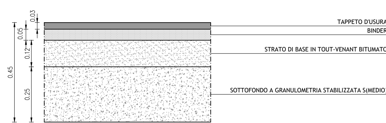
PACCHETTO STRADALE Scale 1:10
