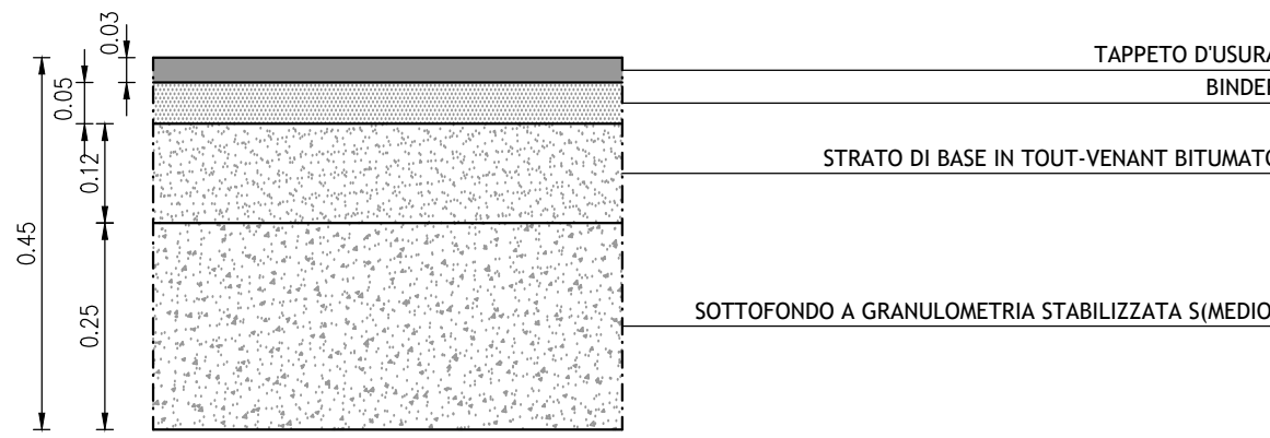
PACCHETTO STRADALE Scale 1:10
