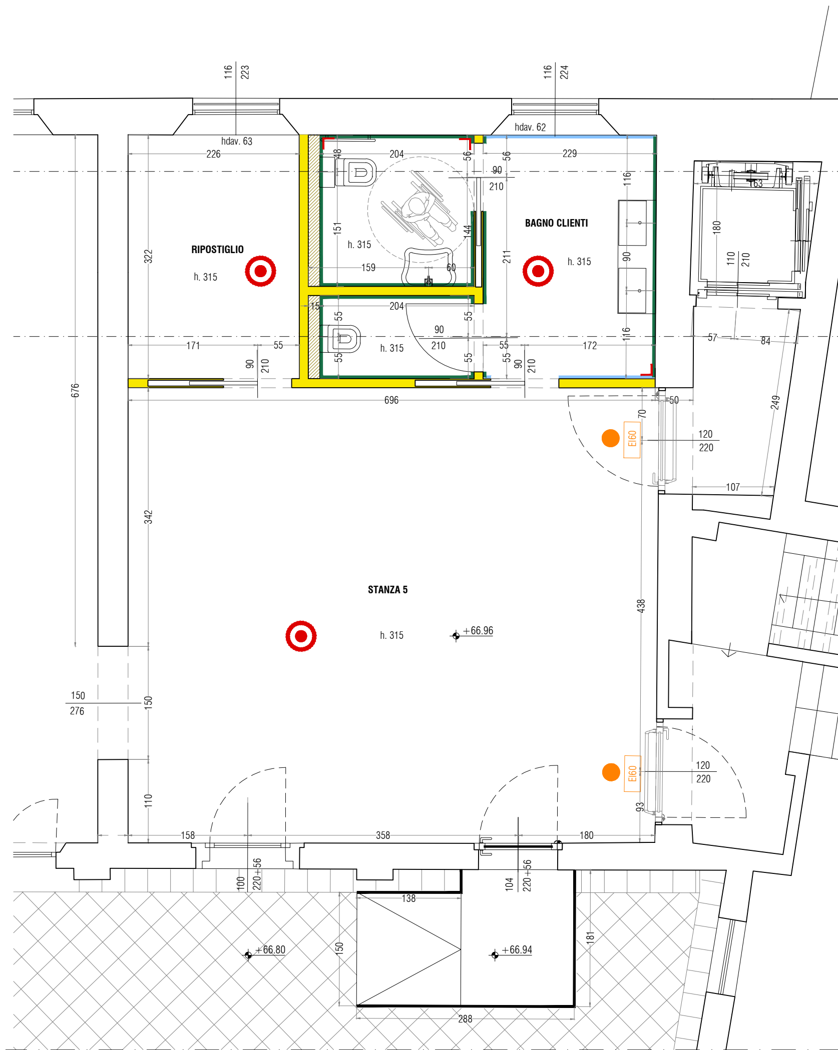
PROGETTO - PIANTA - scala 1:50
