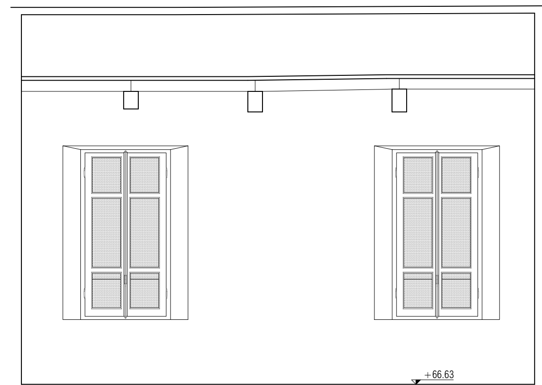
STATO DI FATTO - SEZIONE B - scala 1:50
