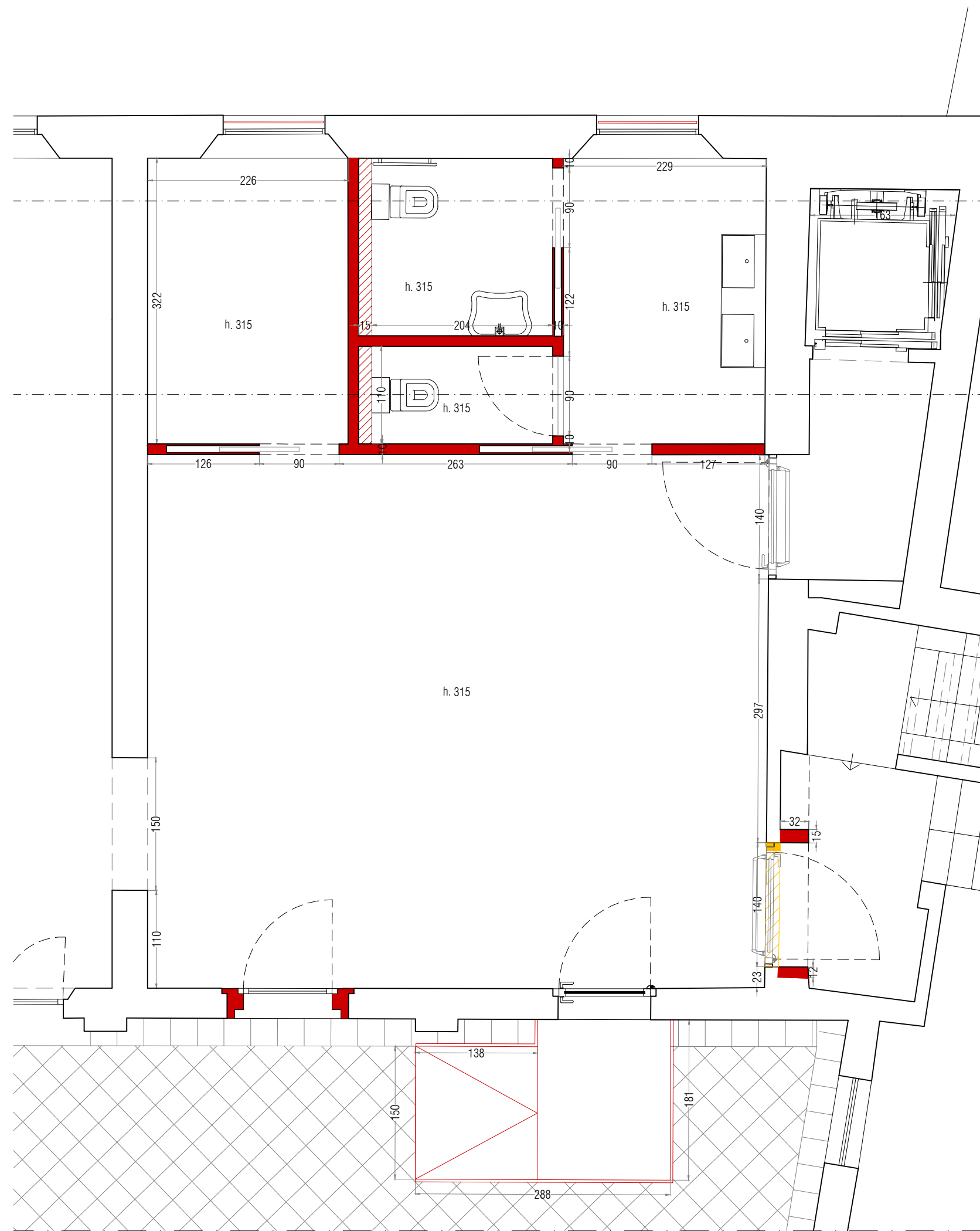
CONFRONTO - PIANTA - scala 1:50
