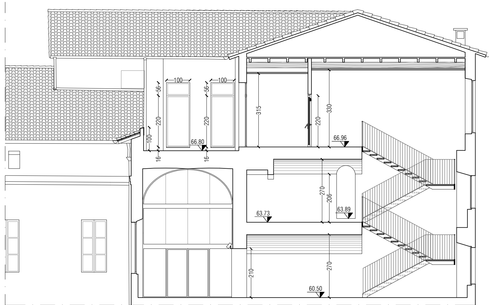
PROGETTO - ESTRATTO SEZIONE H - scala 1:100
