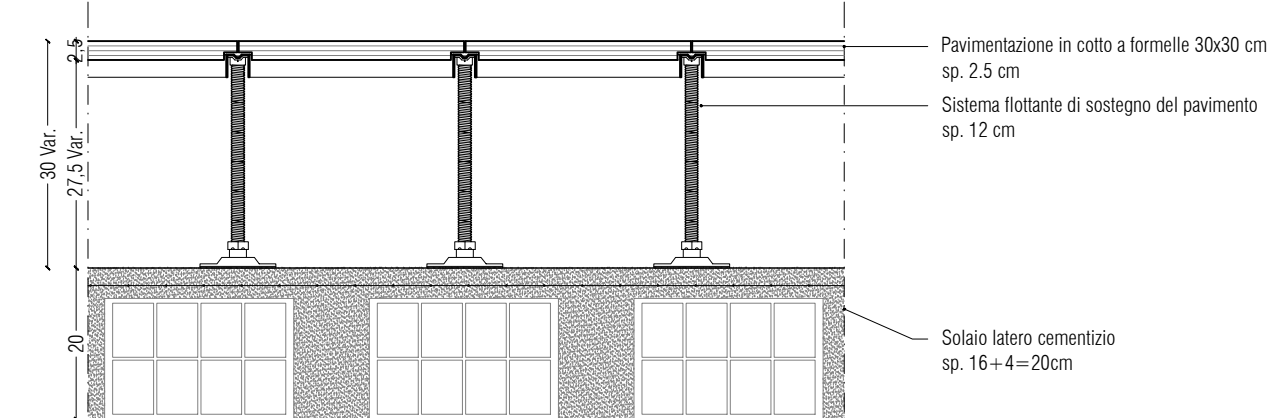
PROGETTO - DETTAGLIO PAVIMENTAZIONE IN COTTO O GRES E NUOVO SOLAIO DI TAMPONAMENTO SCALA - scala 1:10
