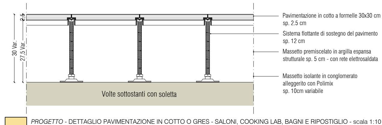
PROGETTO - DETTAGLIO PAVIMENTAZIONE IN COTTO O GRES - SALONI, COOKING LAB, BAGNI E RIPOSTIGLIO - scala 1:10
