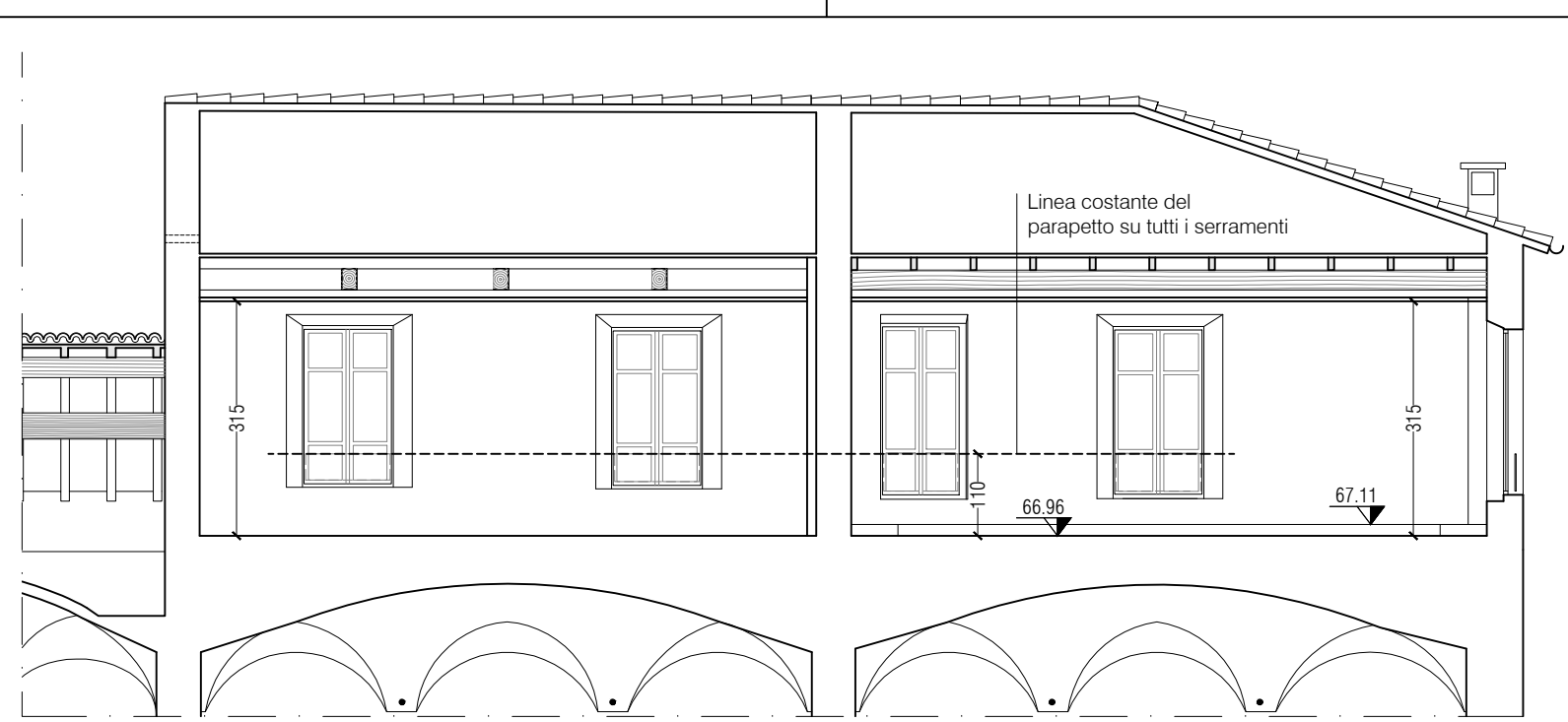
PROGETTO - ESTRATTO SEZIONE C - scala 1:100
