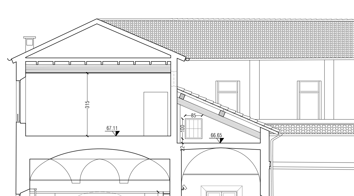
PROGETTO - ESTRATTO SEZIONE E - scala 1:100
