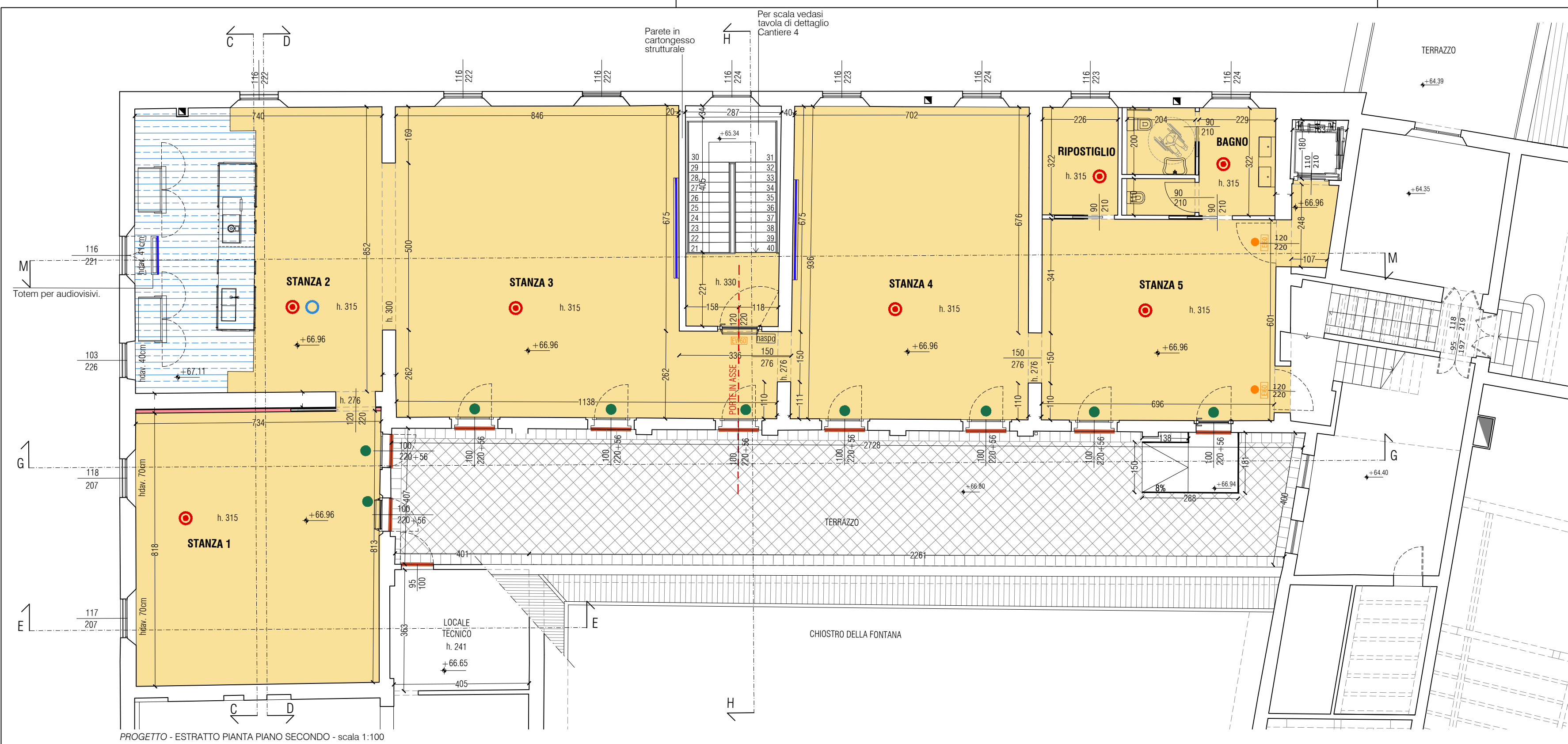
PROGETTO - ESTRATTO PIANTE PIANO SECONDO - scala 1:100
