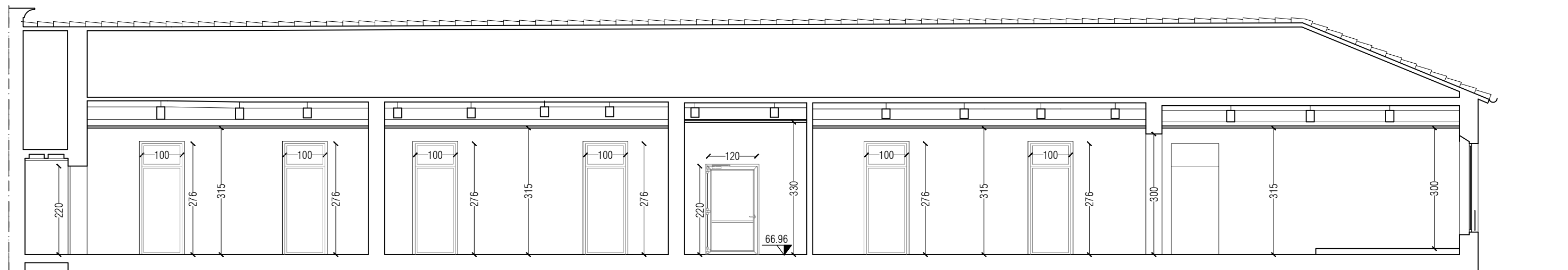
PROGETTO - ESTRATTO SEZIONE M - scala 1:100
