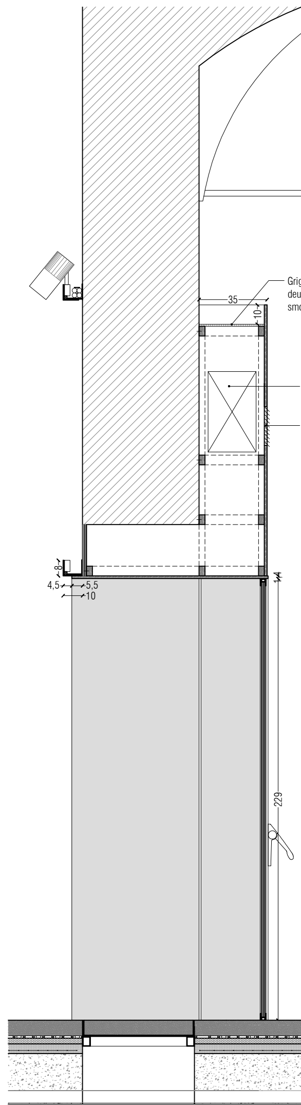
PROGETTO - SEZIONE SERRAMENTO - scala 1:20
