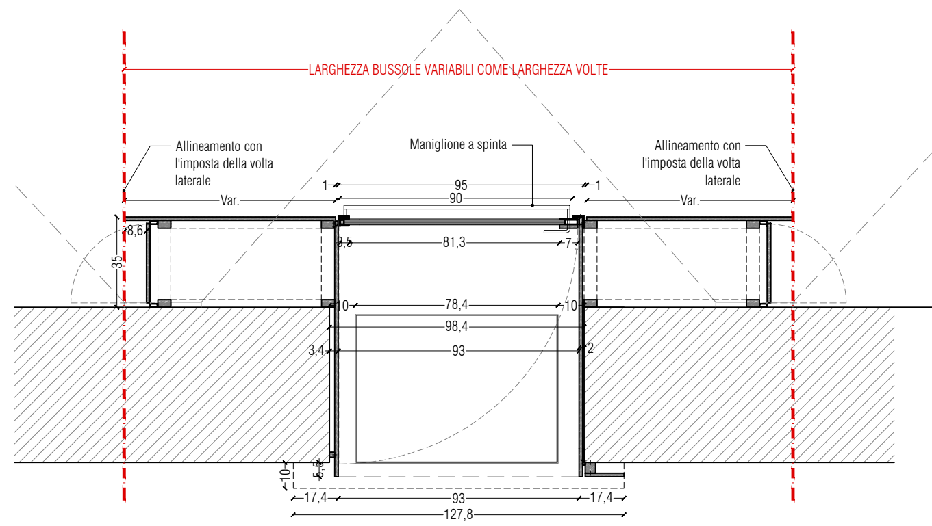
PROGETTO - PIANTA SERRAMENTO - scala 1:20
