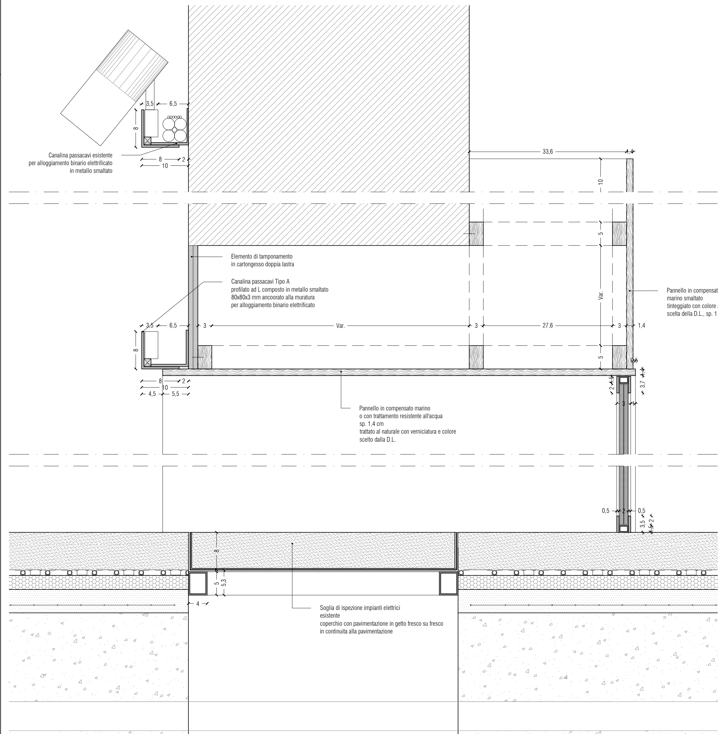
PROGETTO - DETTAGLIO SEZIONE VERTICALE SERRAMENTO - scala 1:5
