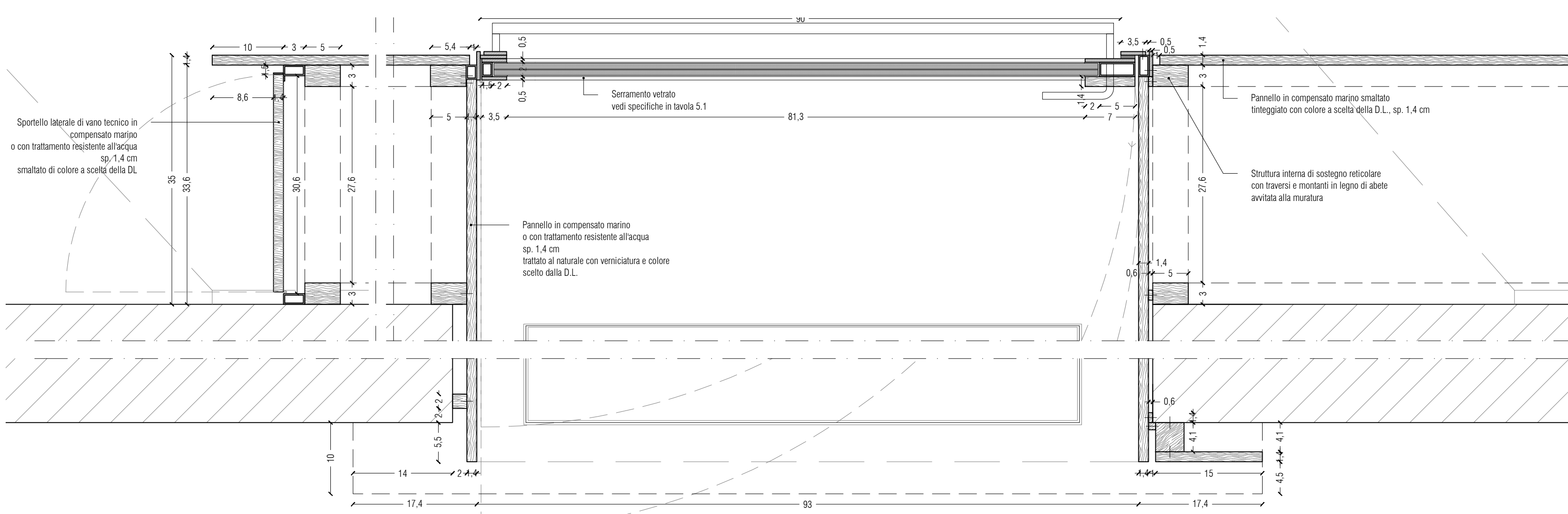
PROGETTO - DETTAGLIO PIANTA SERRAMENTO - scala 1:5
