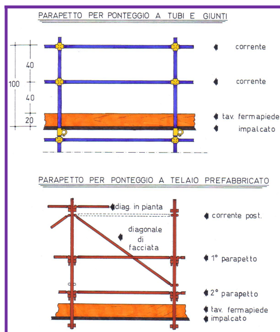
Figura 16. esempi di parapetti
