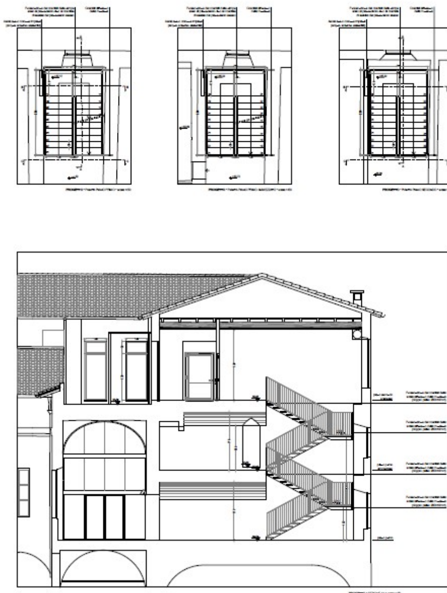
Figura 26: La nuova scala metallica da realizzarsi per collegare il piano primo al piano secondo
