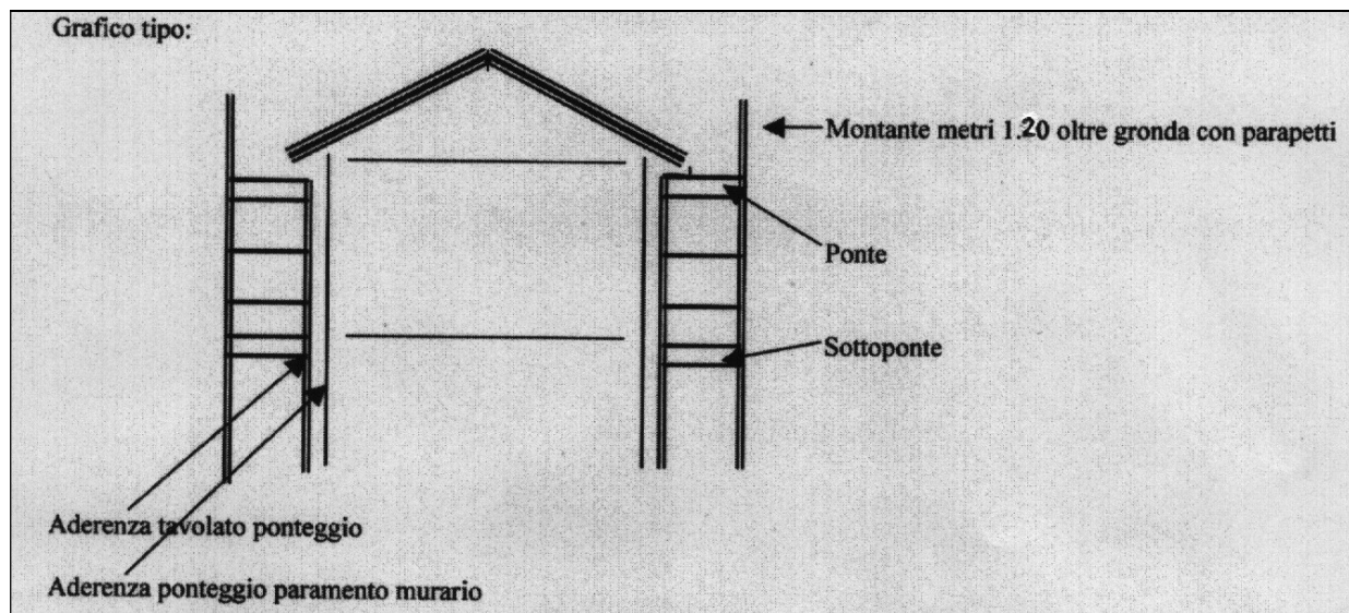
Figura 18. Prescrizioni montaggio ponteggio
