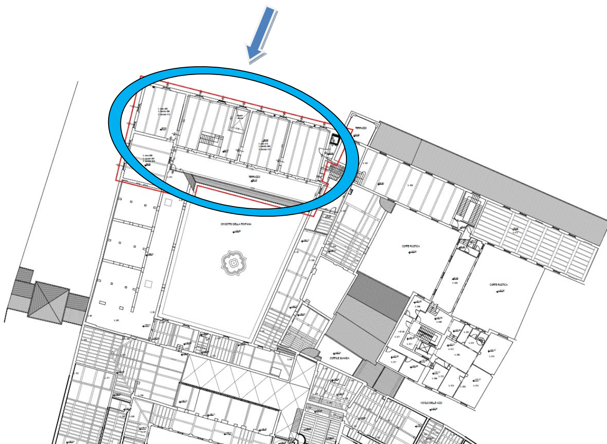
Figura 10 – Pianta del piano secondo con individuazione aree oggetto dell'intervento
