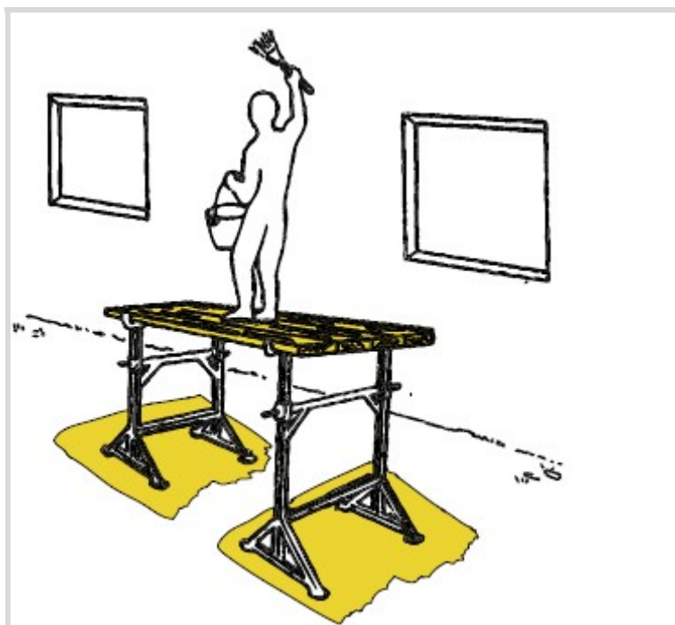
Figura 30: Corretto posizionamento di ponte su cavalletto
