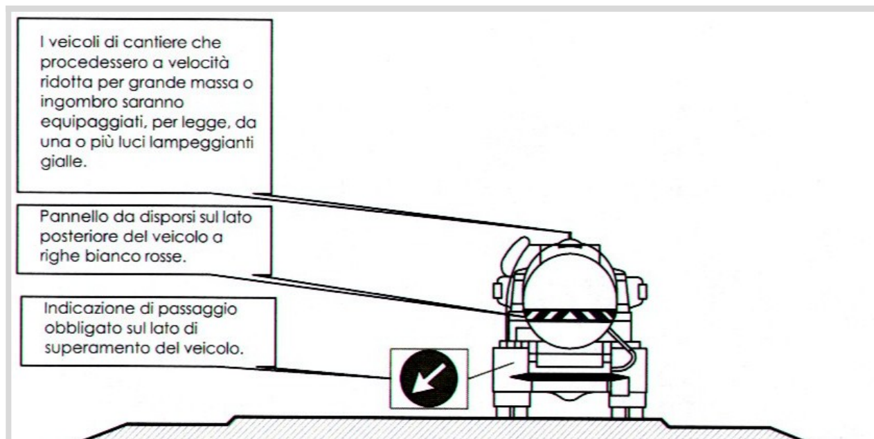
Figura 12. Segnalazione mezzi di cantiere
