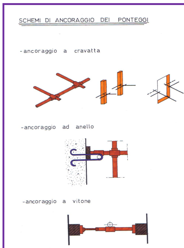
Figura 17. esempi di ancoraggi
