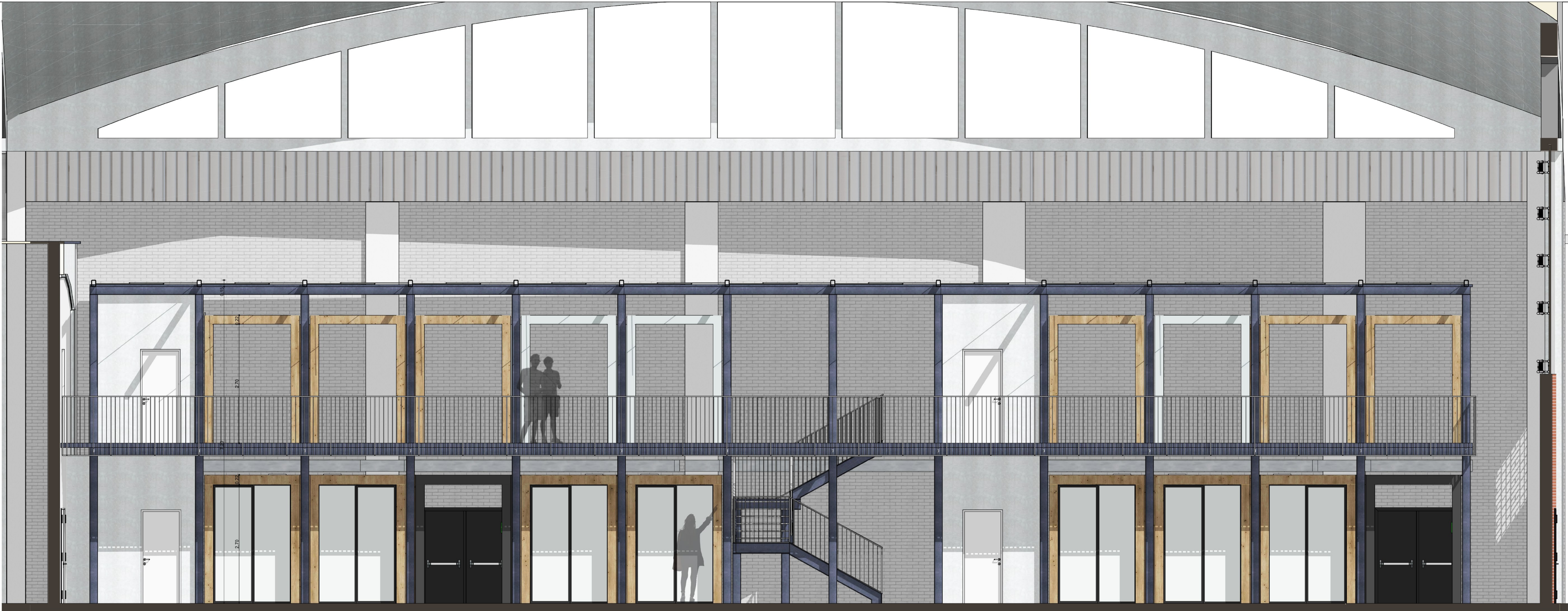
SEZIONE DD scala 1:50
