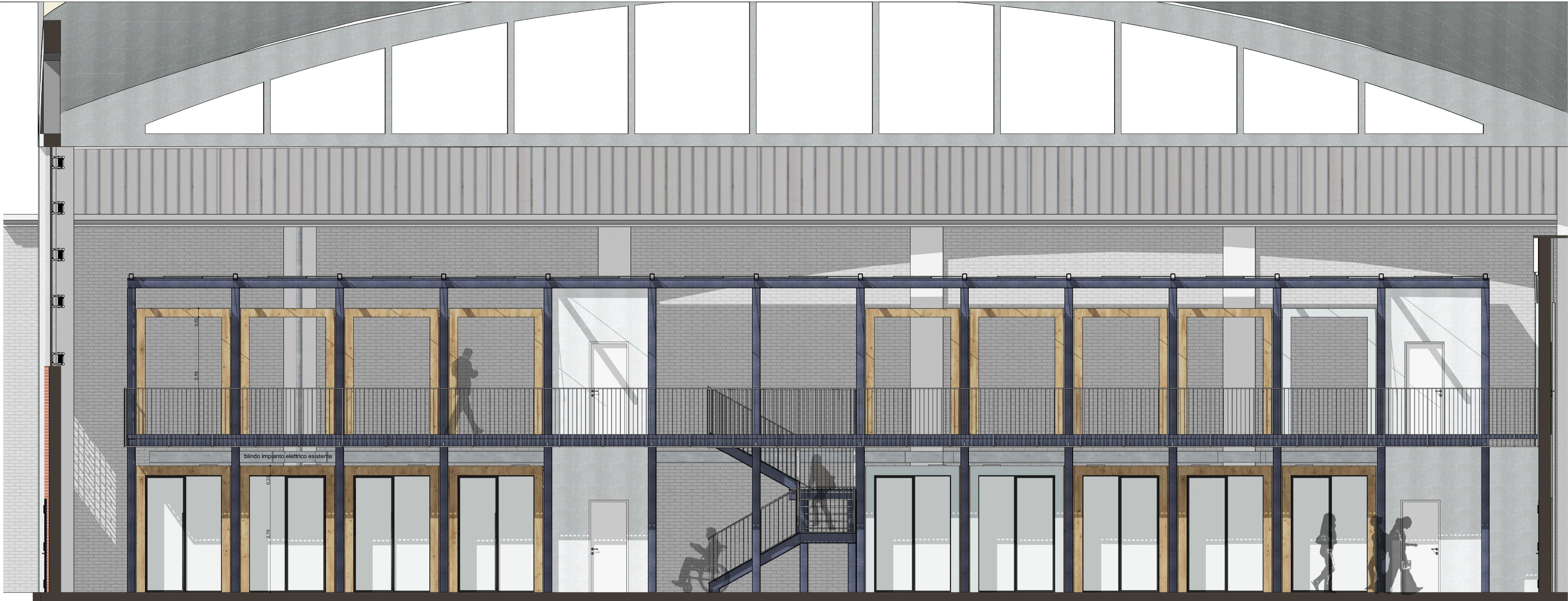
SEZIONE AA scala 1:50
