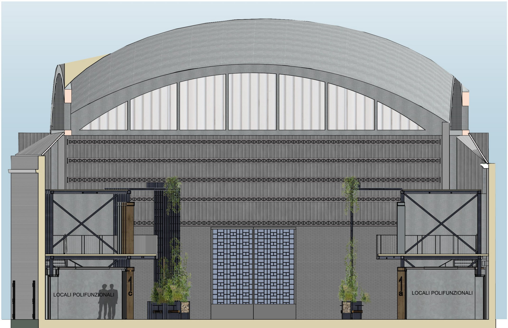
SEZIONE YY scala 1:100
