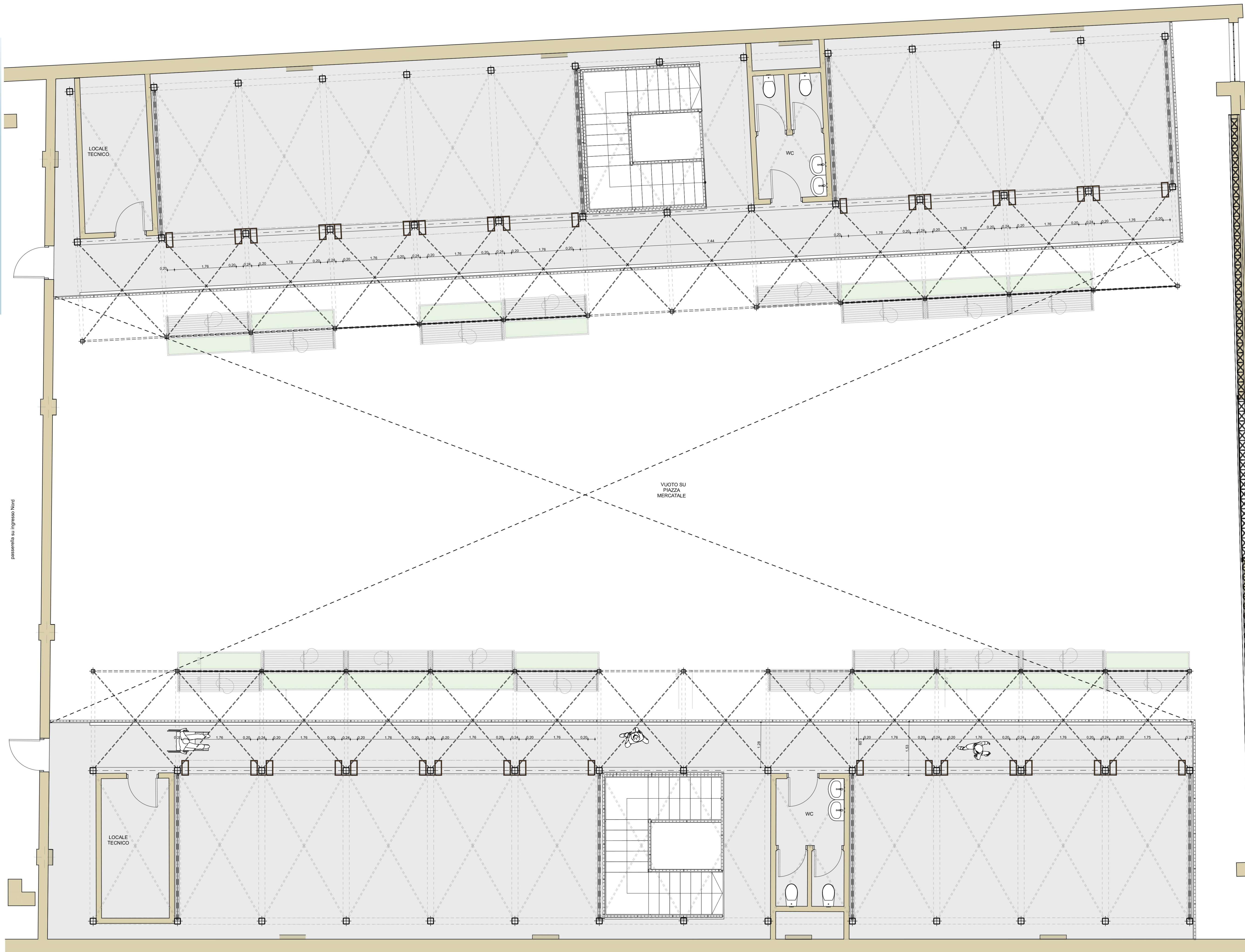
PIANO PRIMO scala 1:50
