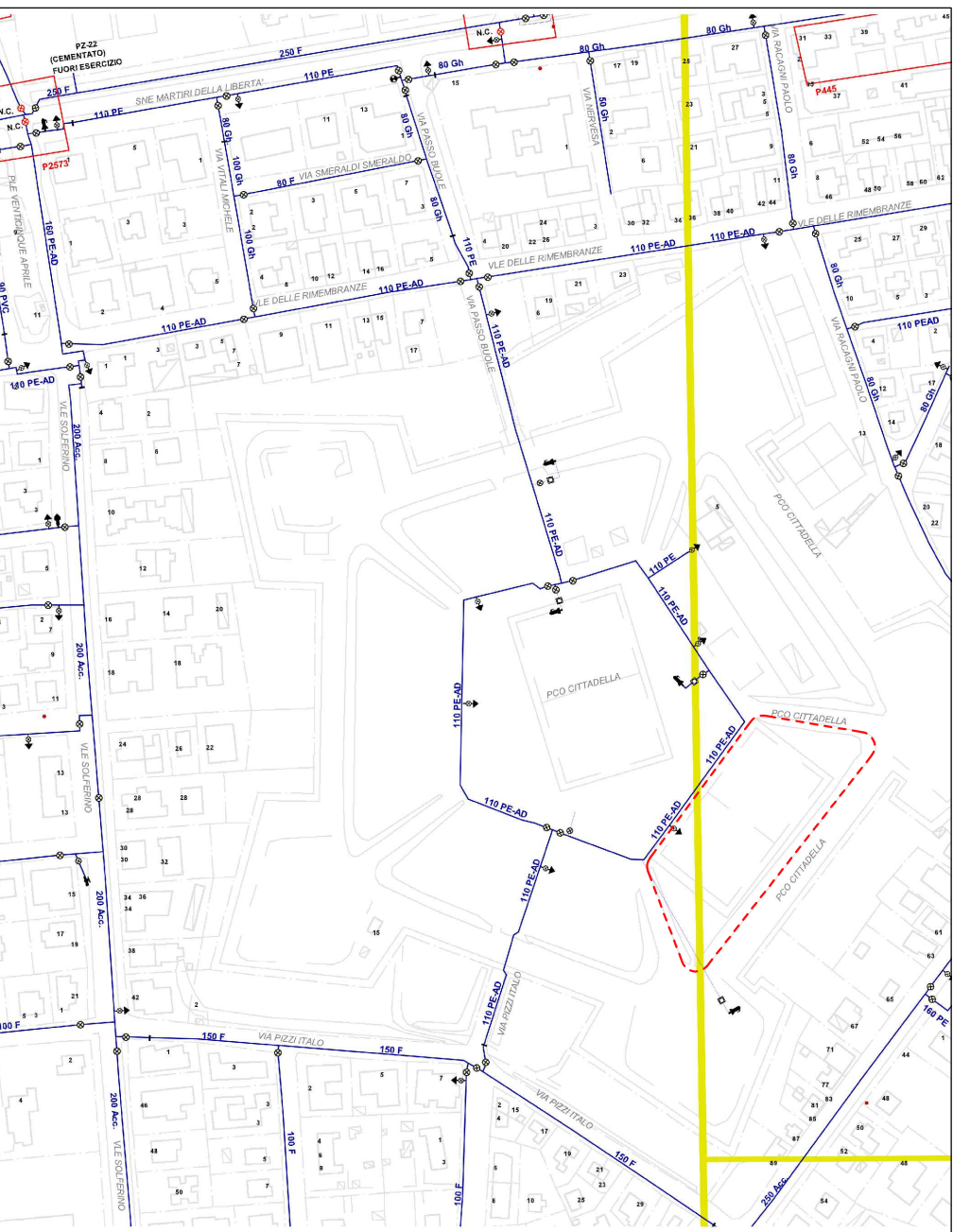
Rete acqua - quadro d'unione
