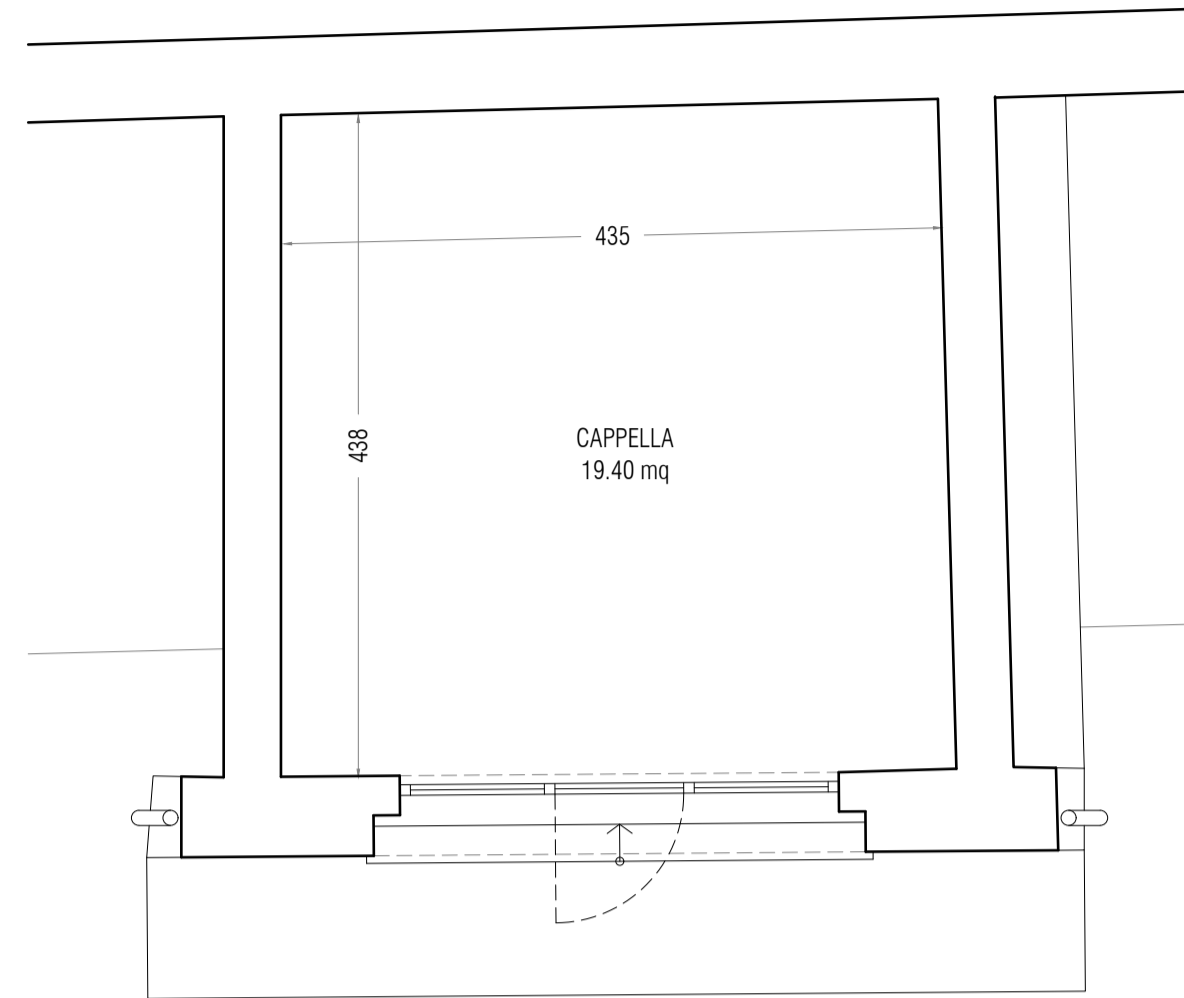
PROGETTO . PIANTA . scala 1:50
