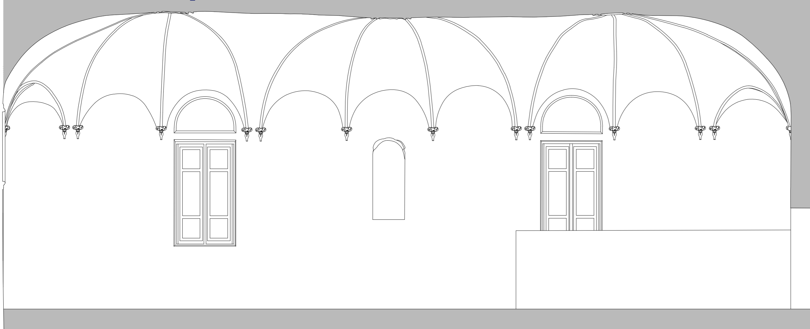
RILIEVO GEOMETRICO E QUADRO FESSURATIVO
