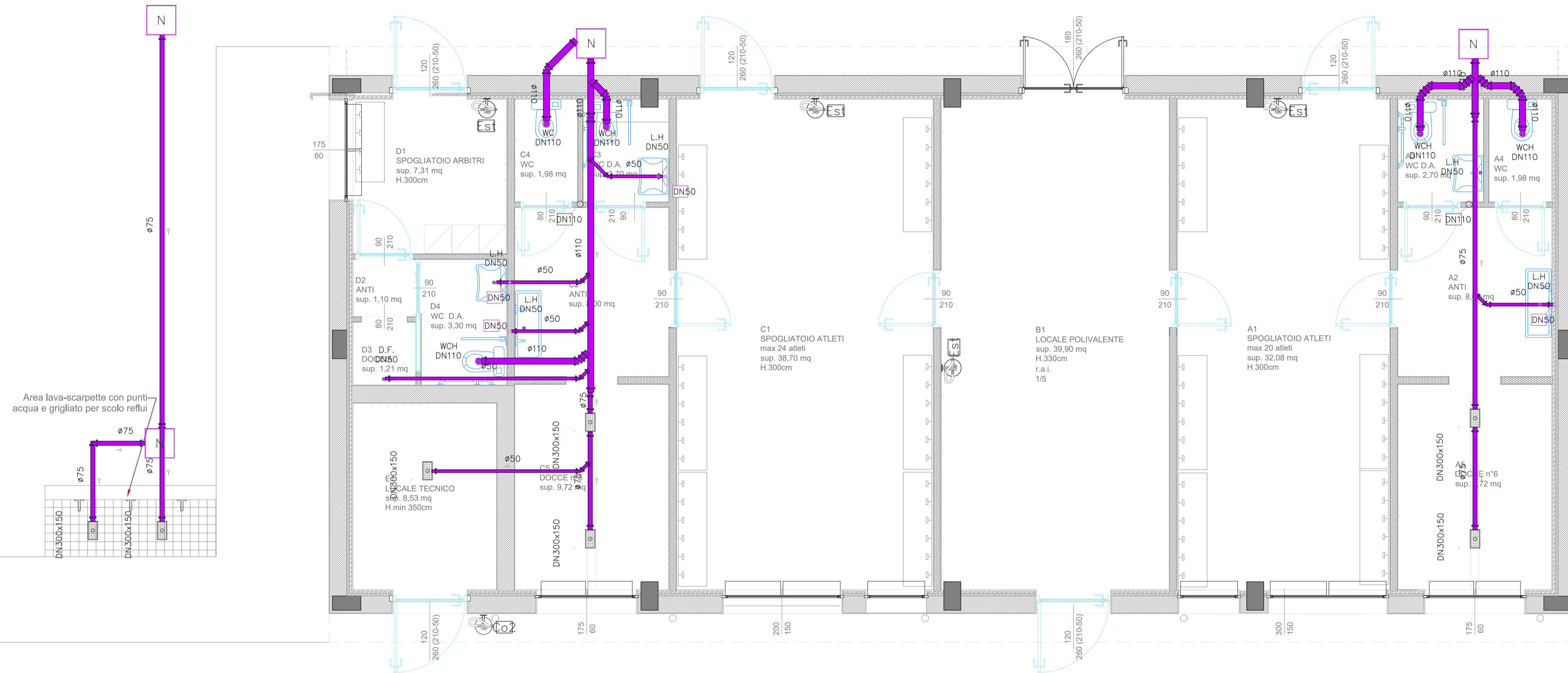
PIANTA (sezione a quota +450 cm.)
