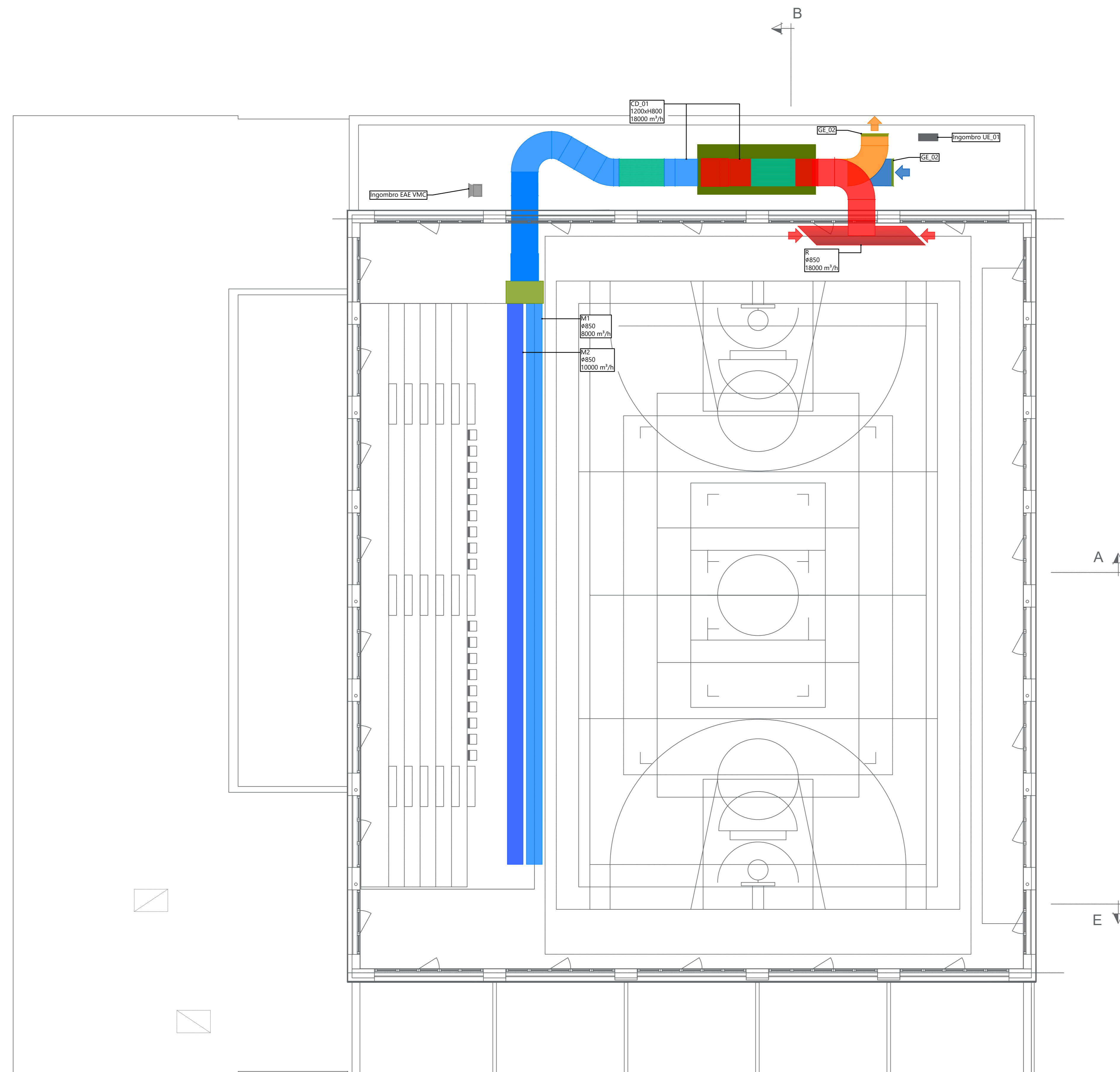
Pianta piano ammezzato (liv. + 5.50)
