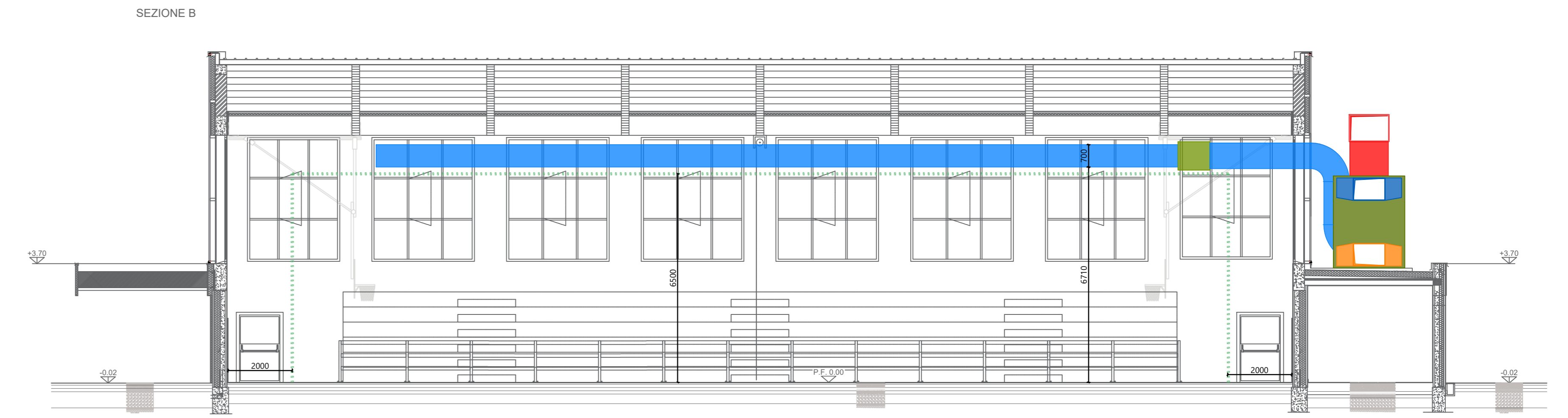
Sezione B
