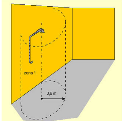
In assenza del piatto doccia la zona 1 è costituita da un solido di forma cilindrica di raggio 0,6 m con il centro sotto al soffione
