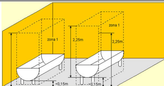
Se il fondo della vasca da bagno o del piatto doccia si trova a più di 0,15 m al di sopra del pavimento, il punto limite di tale zona è situato a 2,25 m al di sopra di questo fondo
