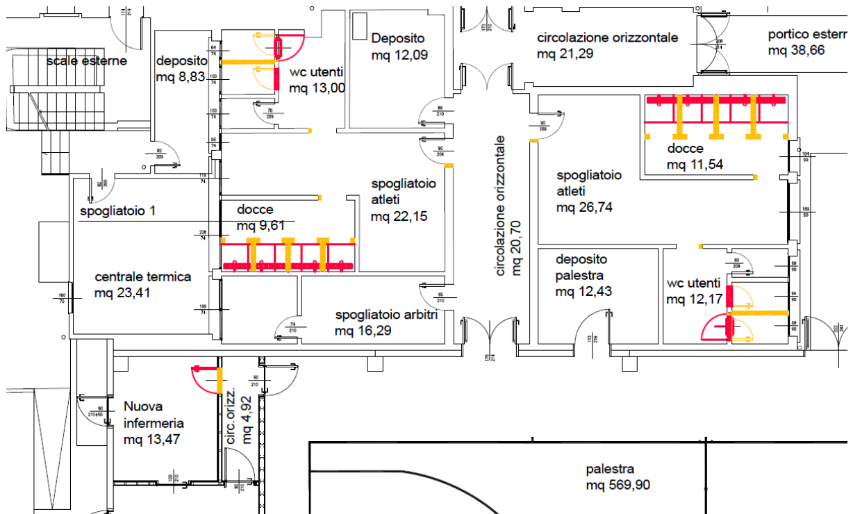
Figura 16 – Tavola di raffronto delle opere edili da eseguirsi negli spogliatoi e nella nuova infermeria
