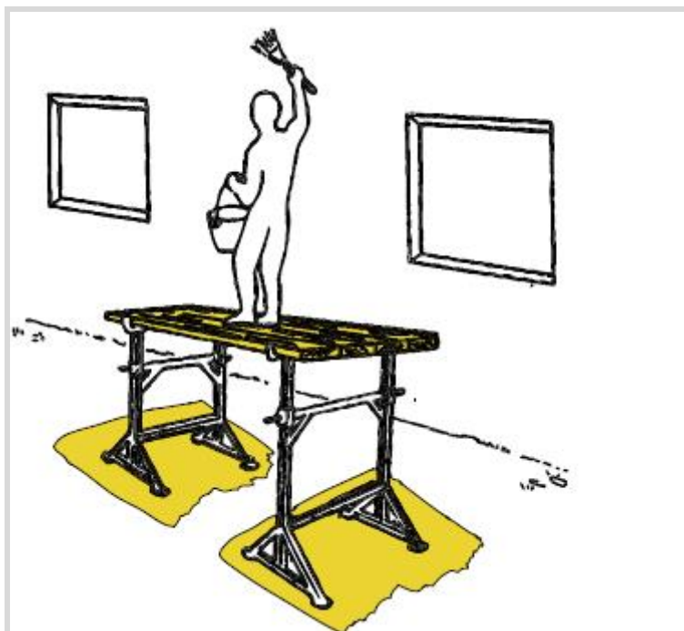
Figura 18 - Corretto posizionamento di ponte su cavalletto
